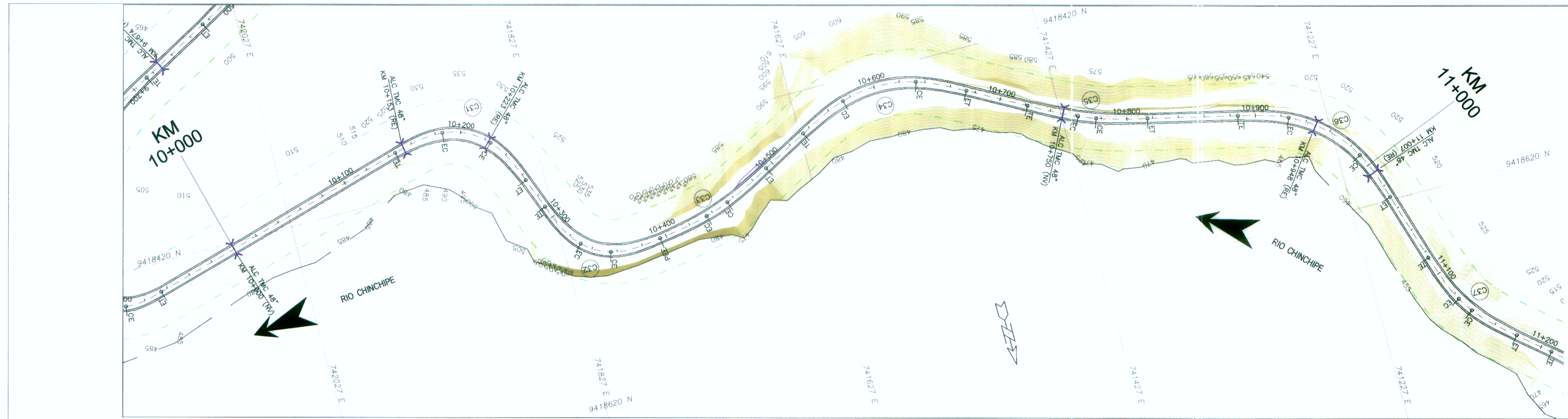
PLANTA 1:2000
