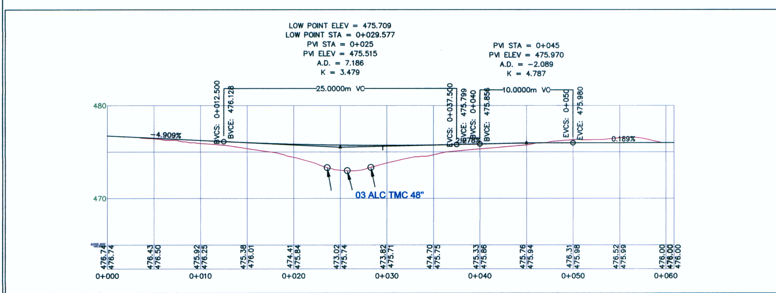
PERFIL LONGITUDINAL ESCALA: 1/ 250
