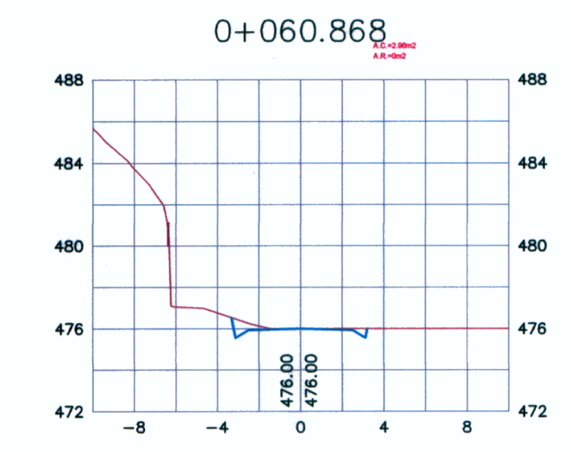
SECCIONES TRANSVERSALES ESCALA: 1/ 250
