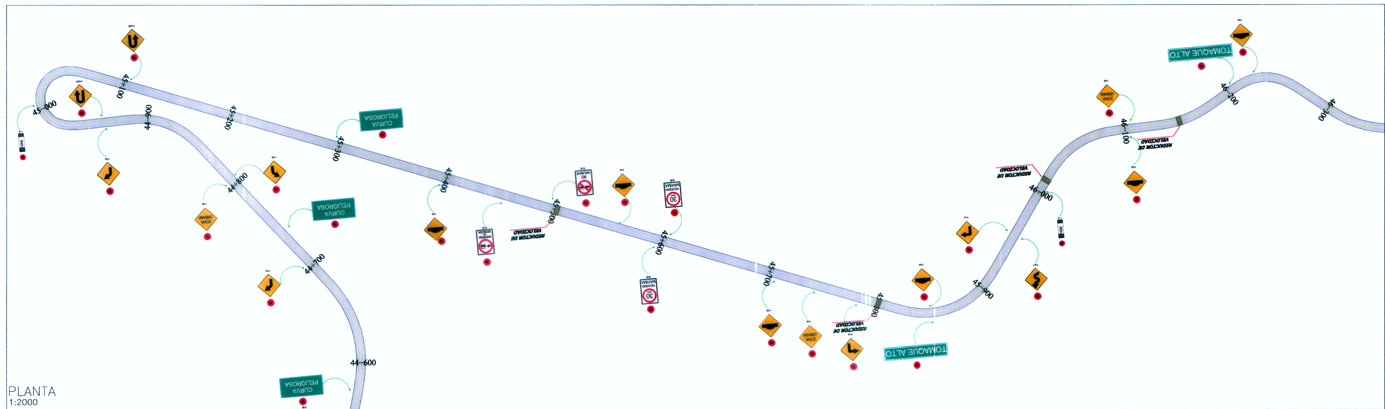
PLANTA 1:2000
