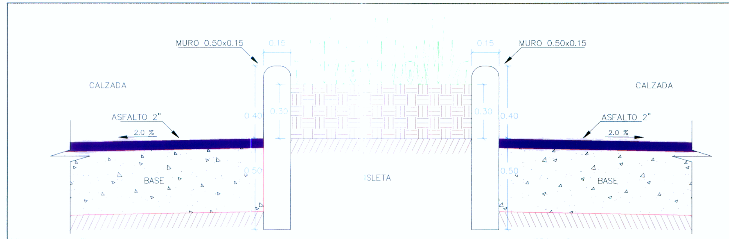
CORTE A-A 1:25
