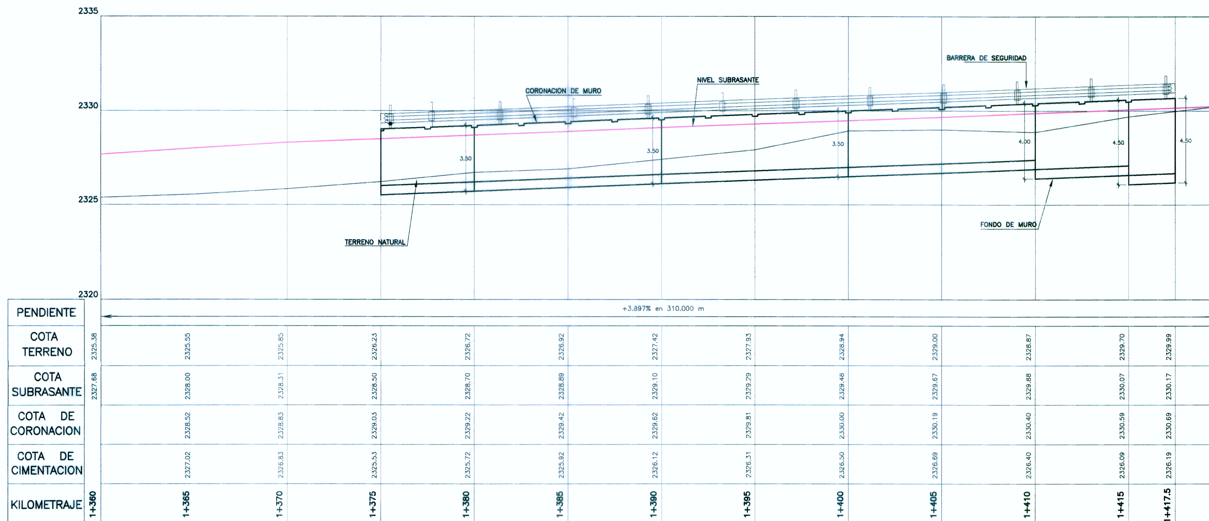
PERFIL LONGITUDINAL (VIA PROYECTADA)
