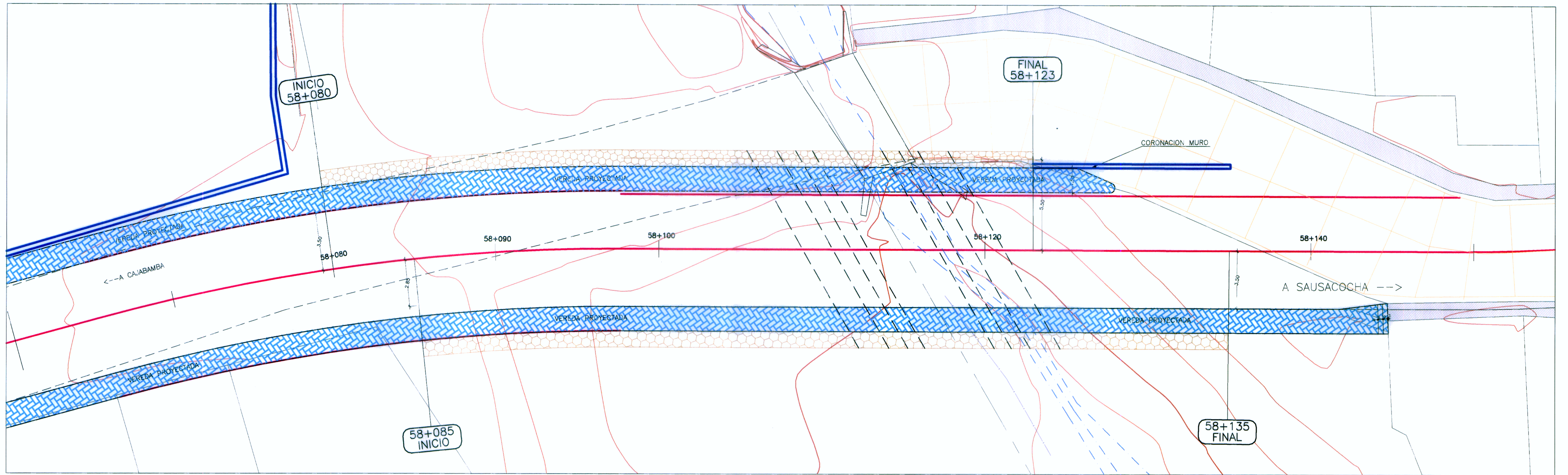
PLANTA ESC.: 1/125
