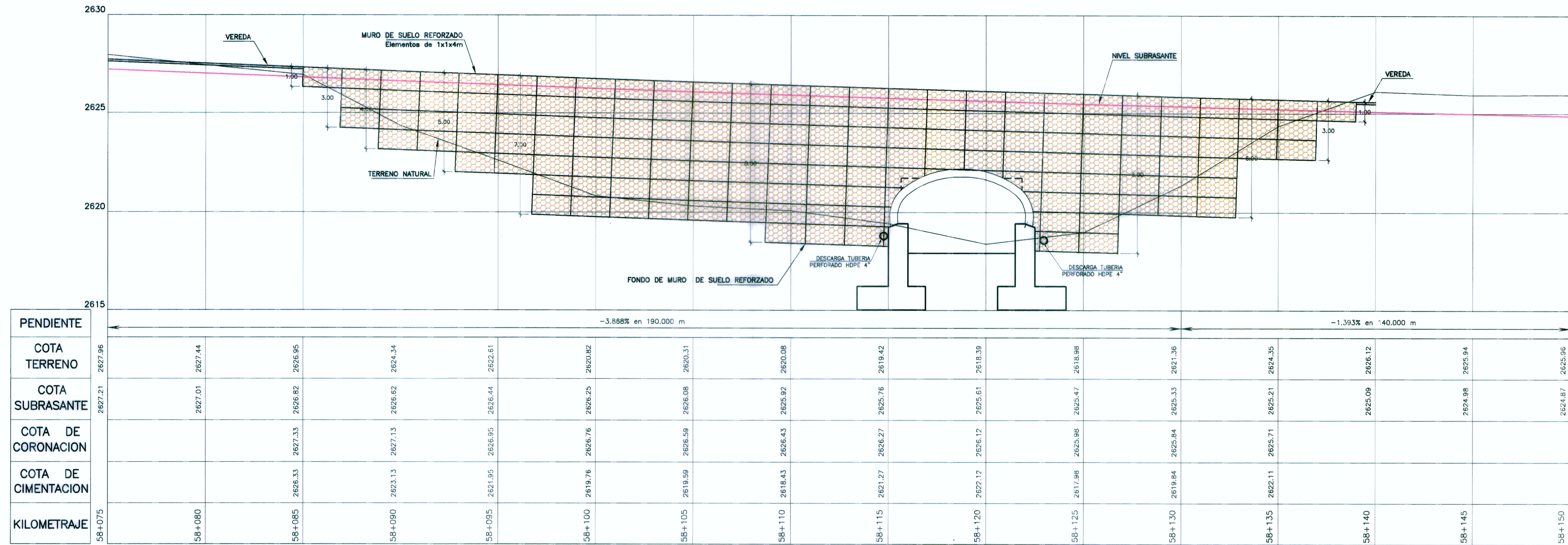
PERFIL LONGITUDINAL LADO DERECHO
