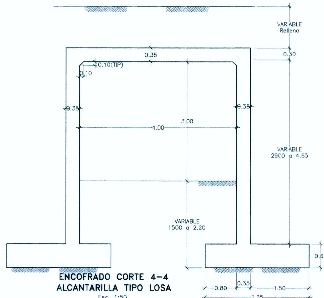
ENCOFRADO ALCANTARILLA TIPO LOSA Esc. 1:50
