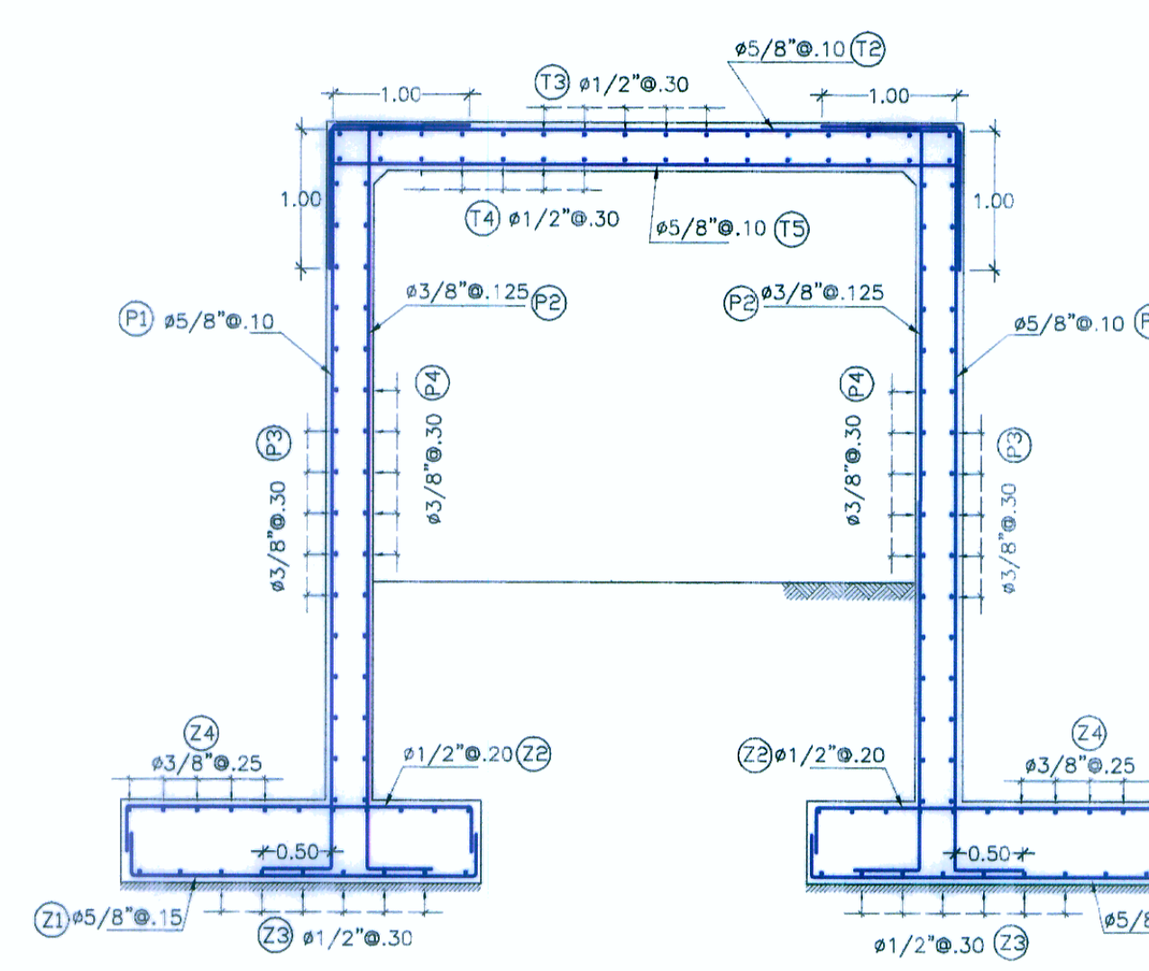
ARMADURA CORTE 4-4 Esc. 1:50
