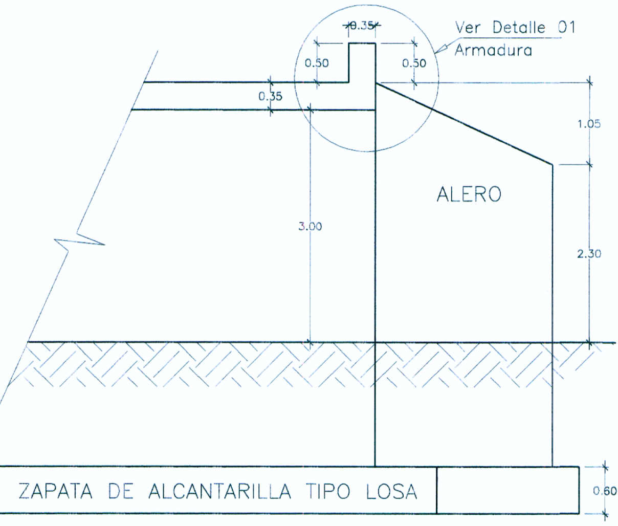
CORTE 2-2 ALCANTARILLA TIPO LOSA Esc. 1:50
