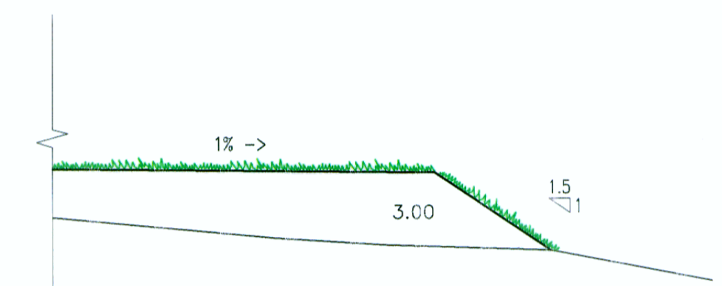
SECCION TIPICA DE BANQUETA 1:200
