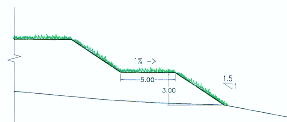
SECCION TIPICA DE BANQUETA
