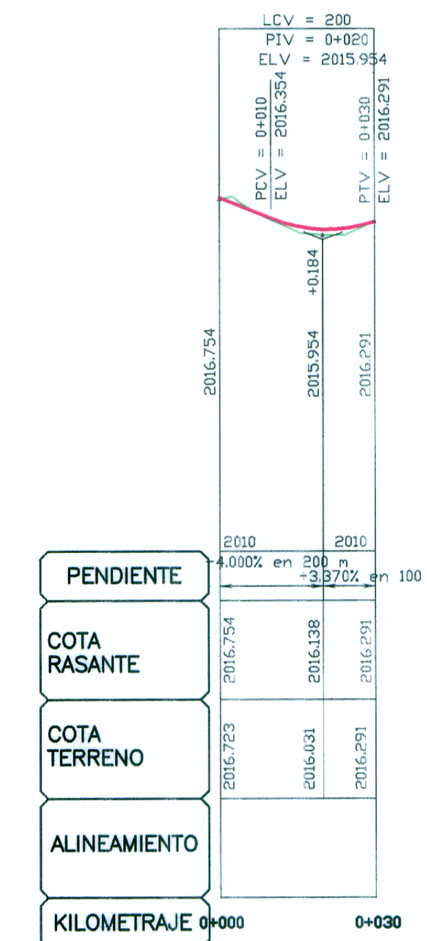
PERFIL 1:1000
