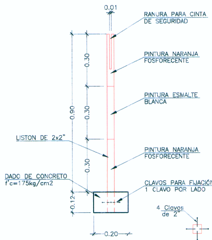
POSICION DE CLAVOS
