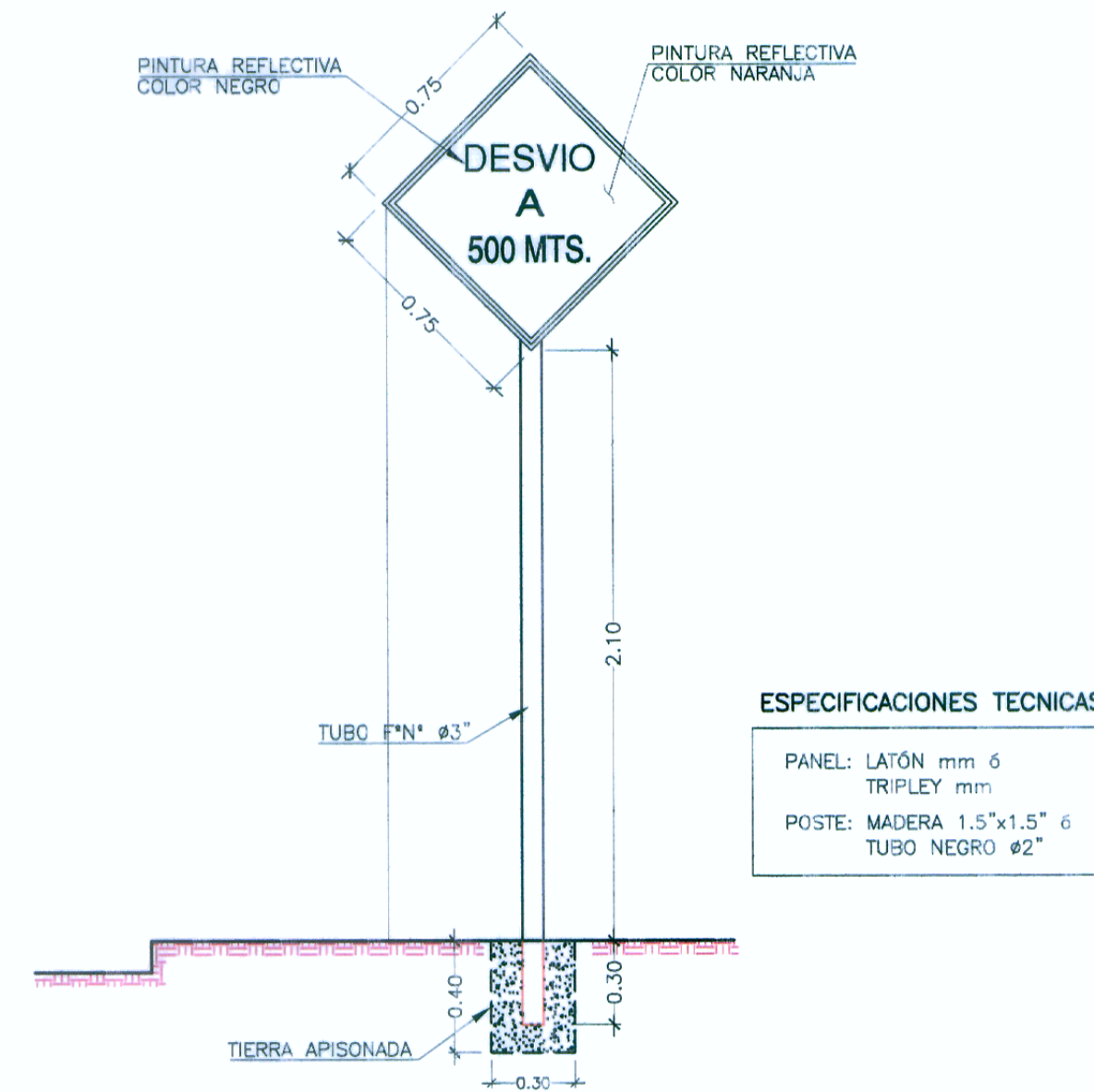
ELEVACION FRONTAL SEÑALES UNIPOSTE ESC. 1/25
