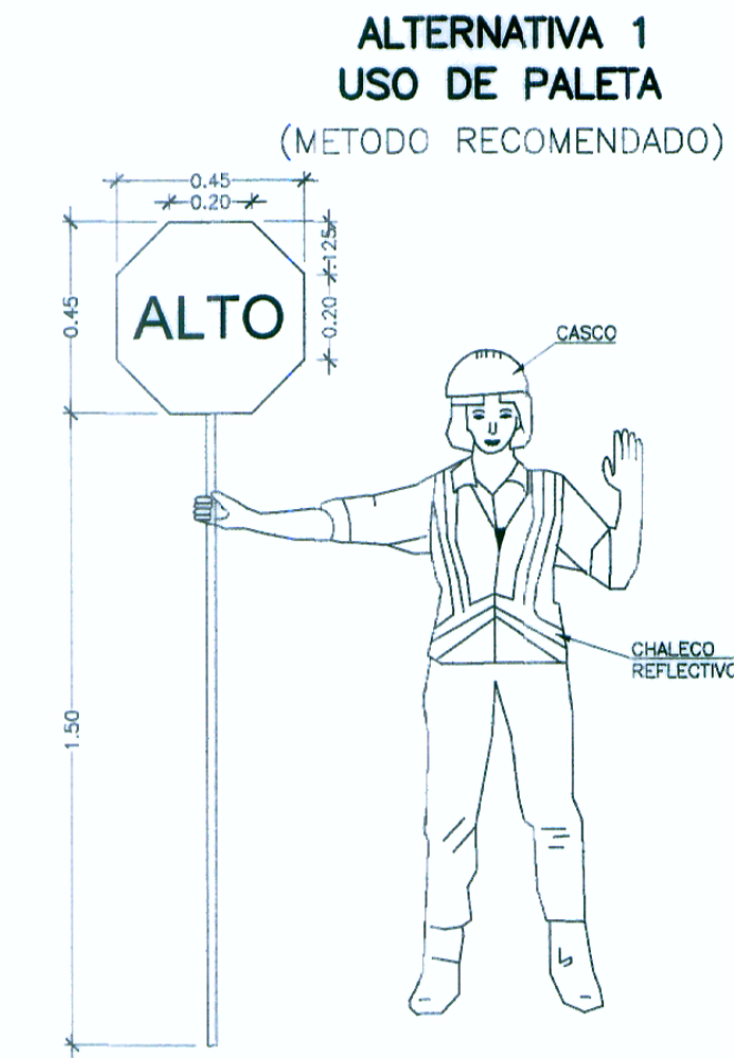
ALTO
