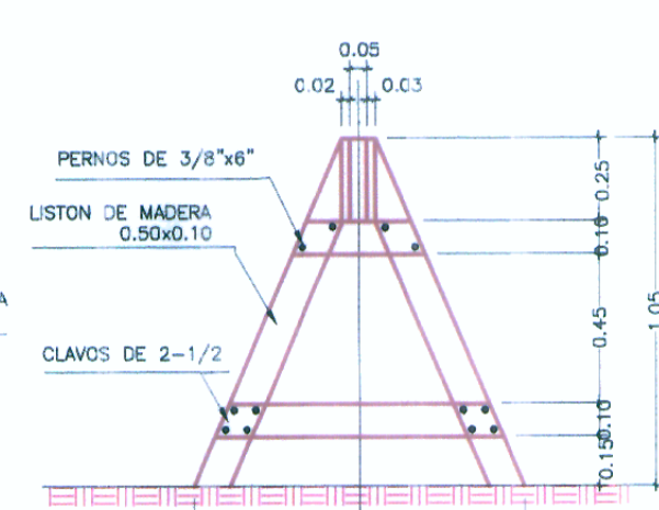
ELEVACION LATERAL
