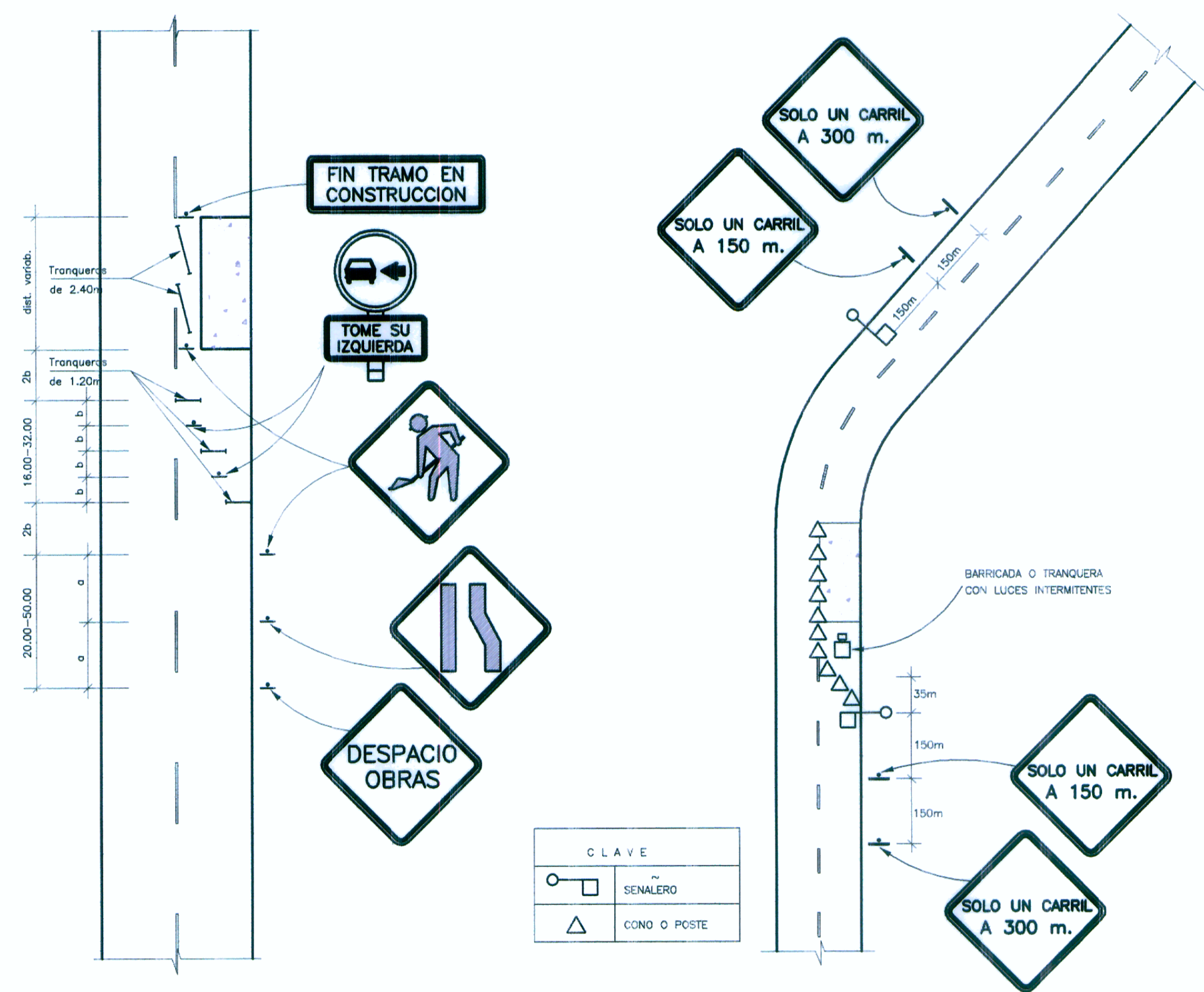
SEÑALIZACION EN ZONA DE TRABAJO ESC. 1/25
