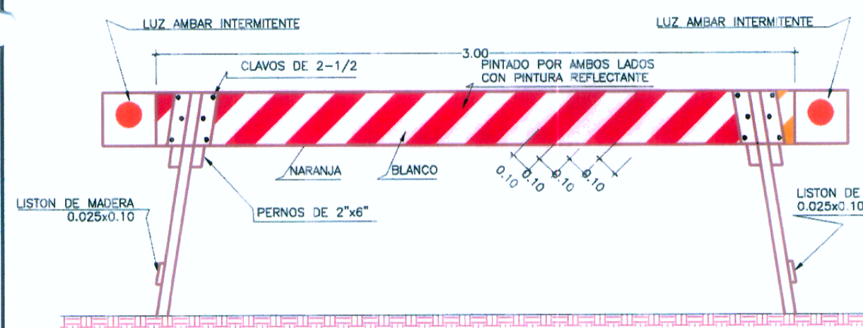
ELEVACION FRONTAL
