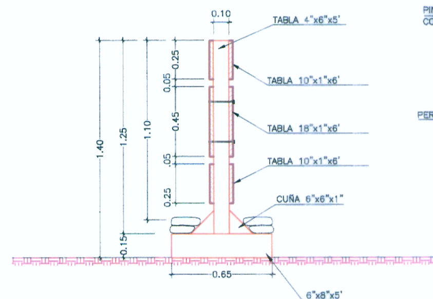
ELEVACION LATERAL ESC. 1/25
