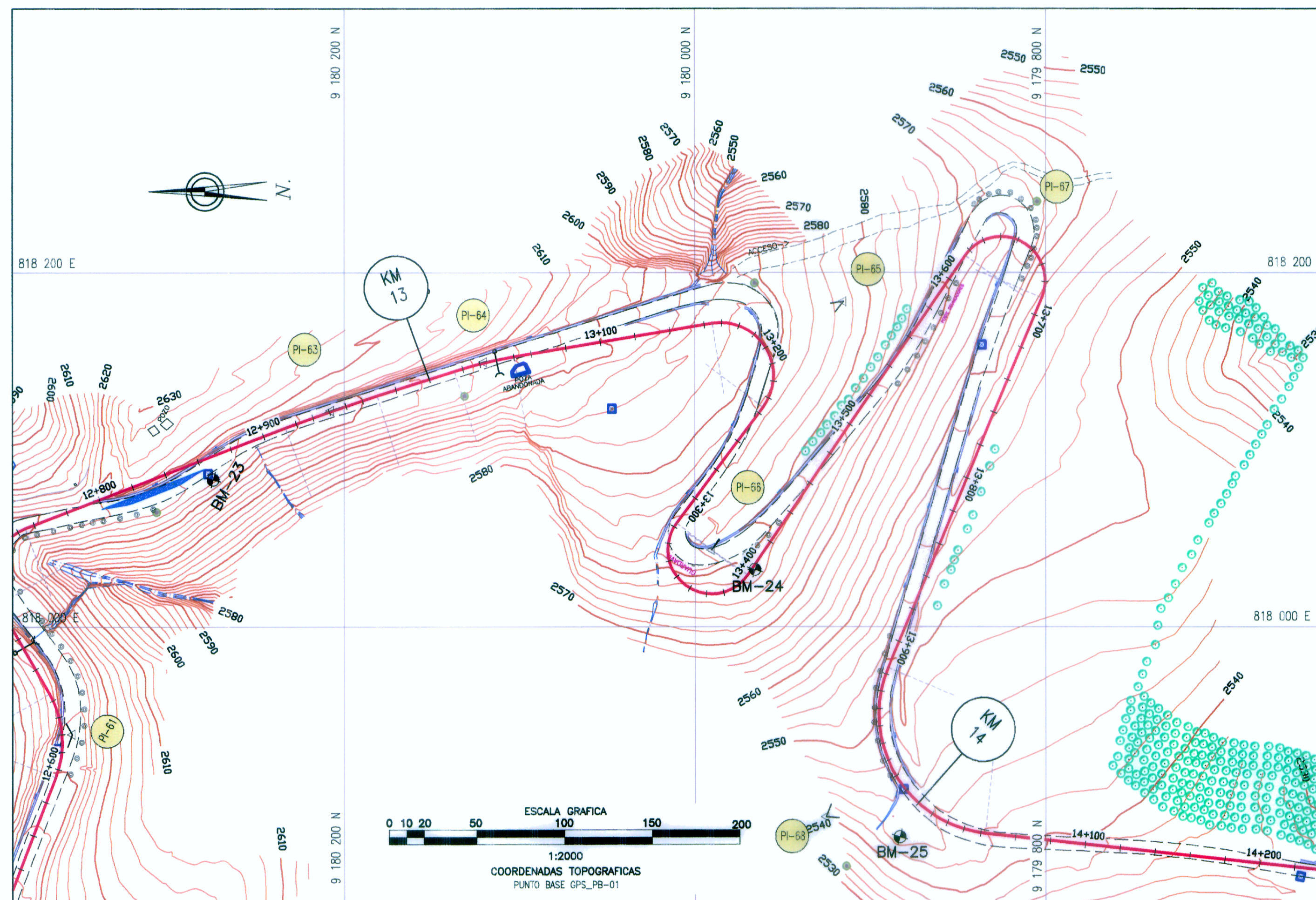
PLANTA 1:2000
