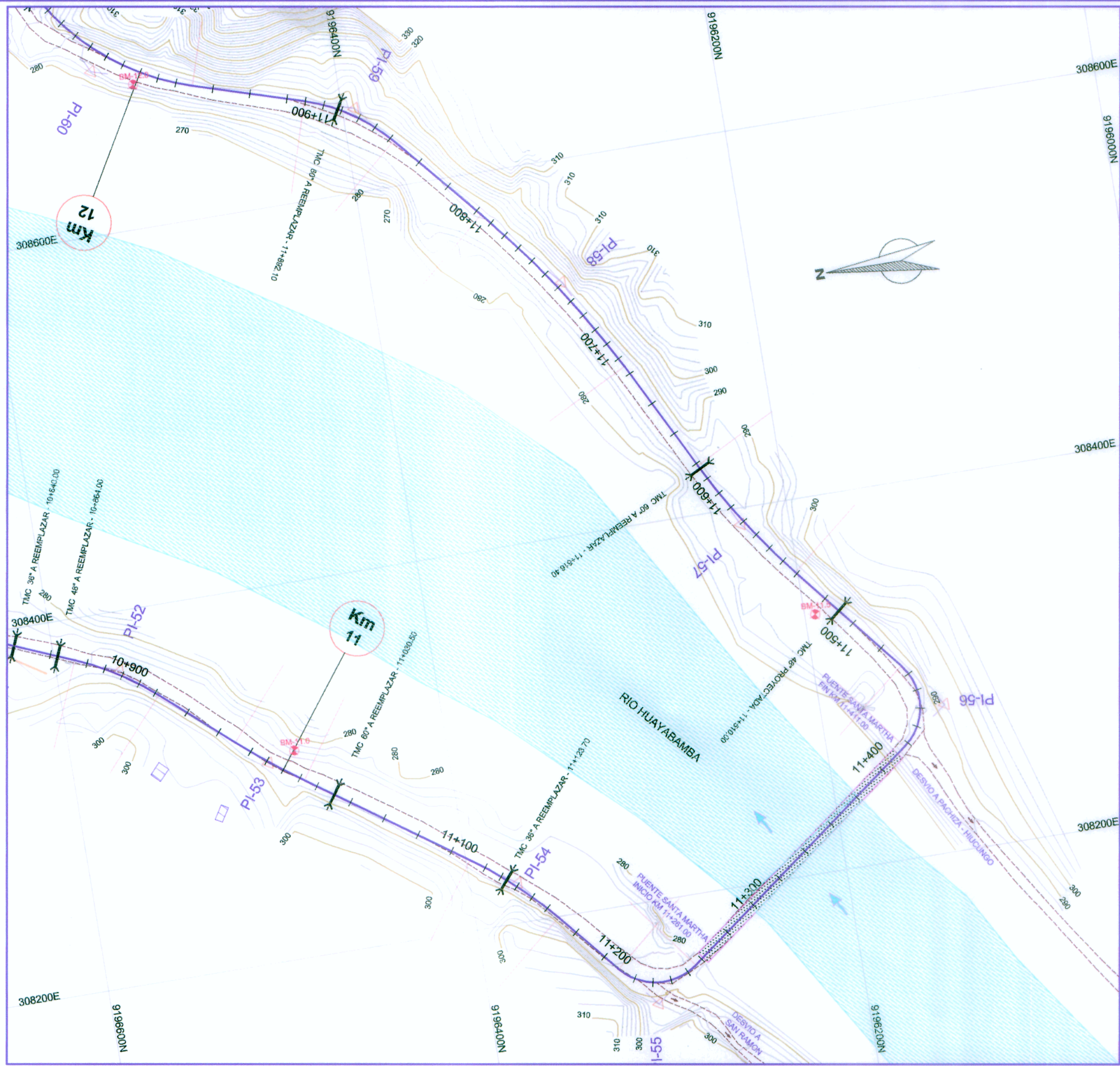
PLANTA ESCALA 1/2000
