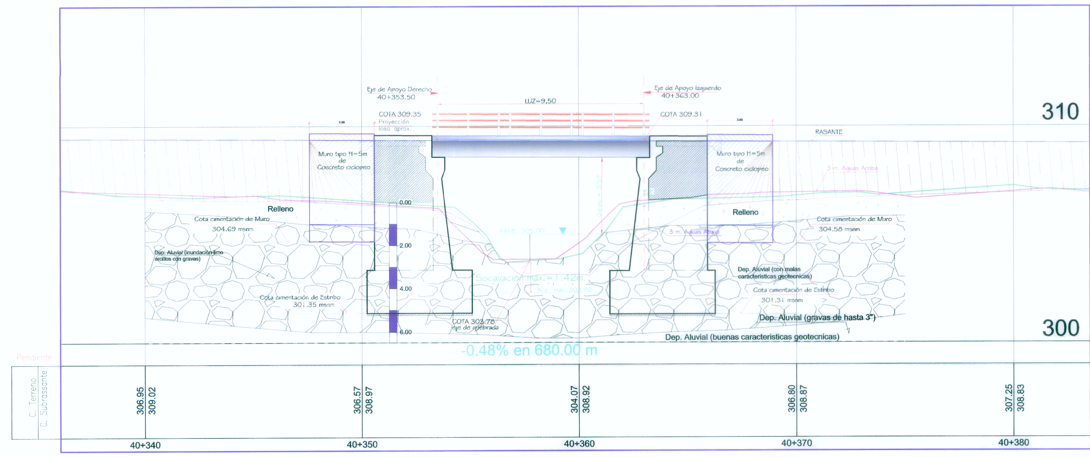
ELEVACIÓN Esc. 1/100
