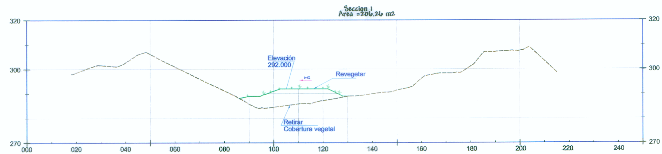
Secciones Transversales esc 1/750
