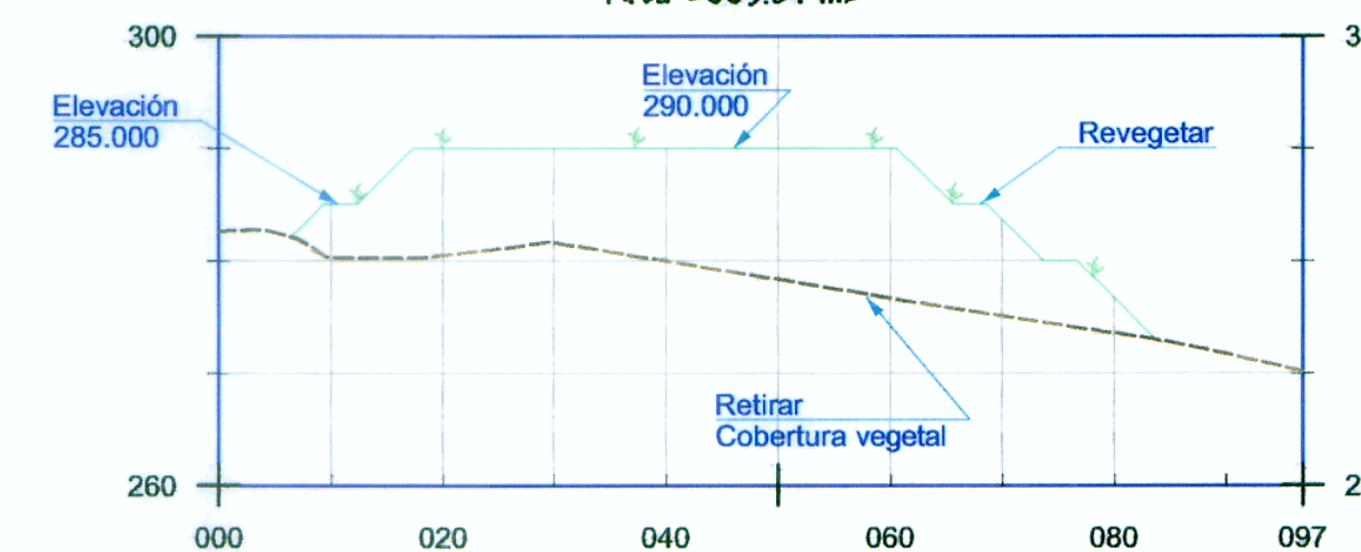
Sección 1 Área = 665.84 m 2
