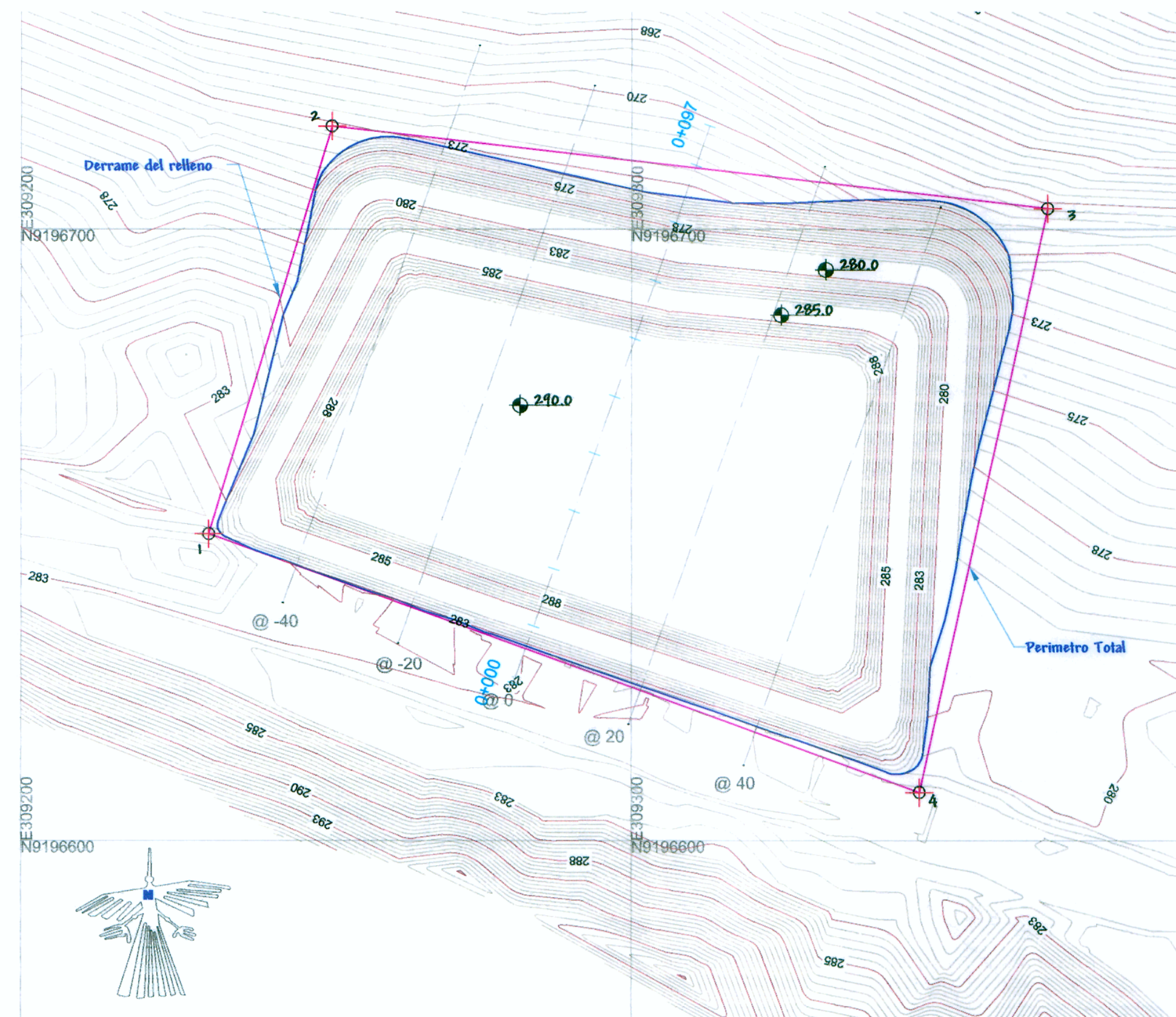
DME N° 04 - km. 12+700 esc 1/750
