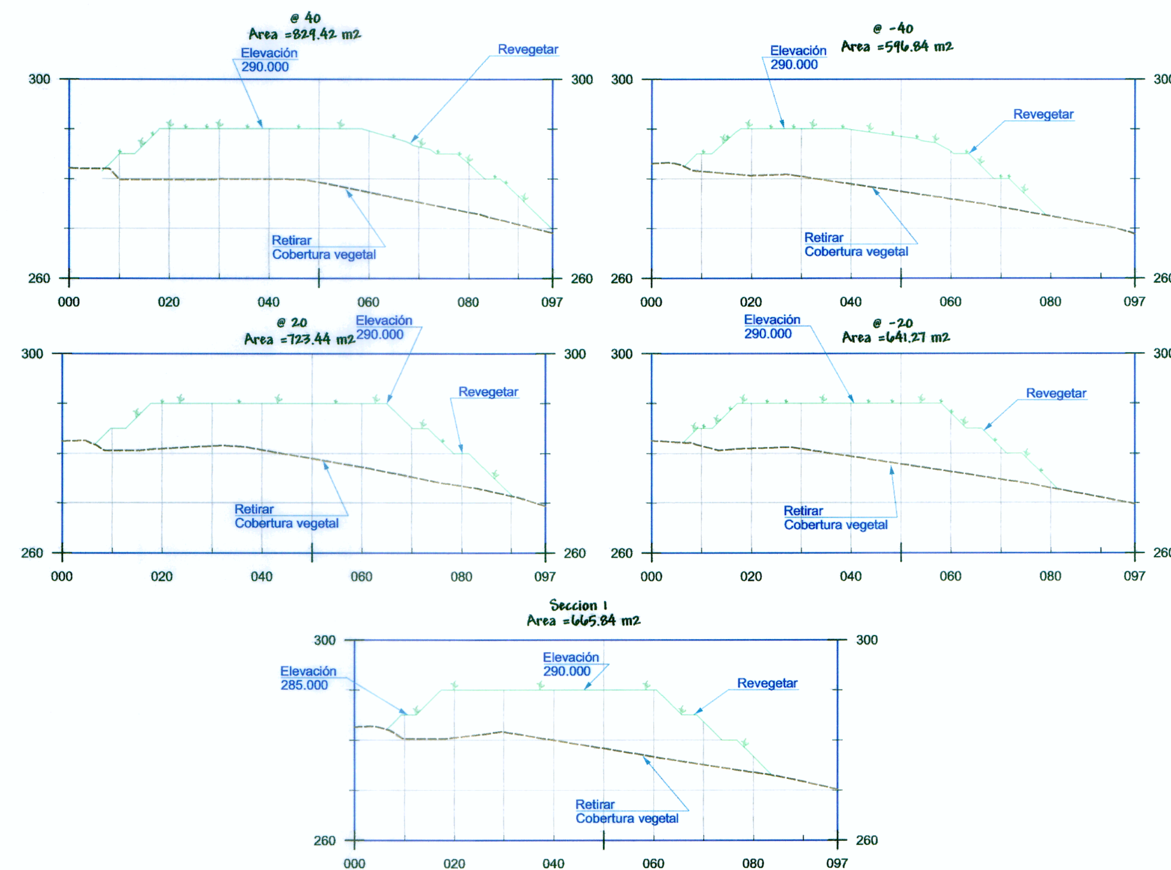
Secciones Transversales esc 1/750
