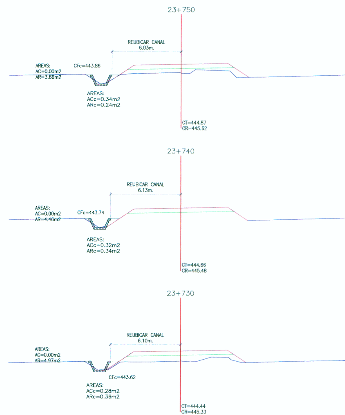
SECCIONES ESC.: A1: 1/200 A3: 1/100 CANAL REUBICADO TRAMO: Km.23+580 - Km.23+750 LONGITUD: 170 m.
