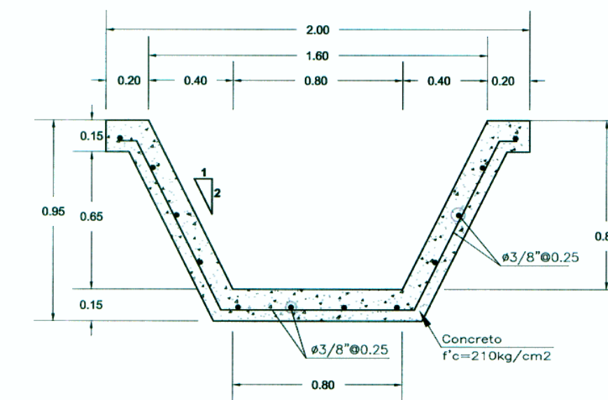
ESPECIFICACIONES TECNICAS CANAL TRAPEZOIDAL
