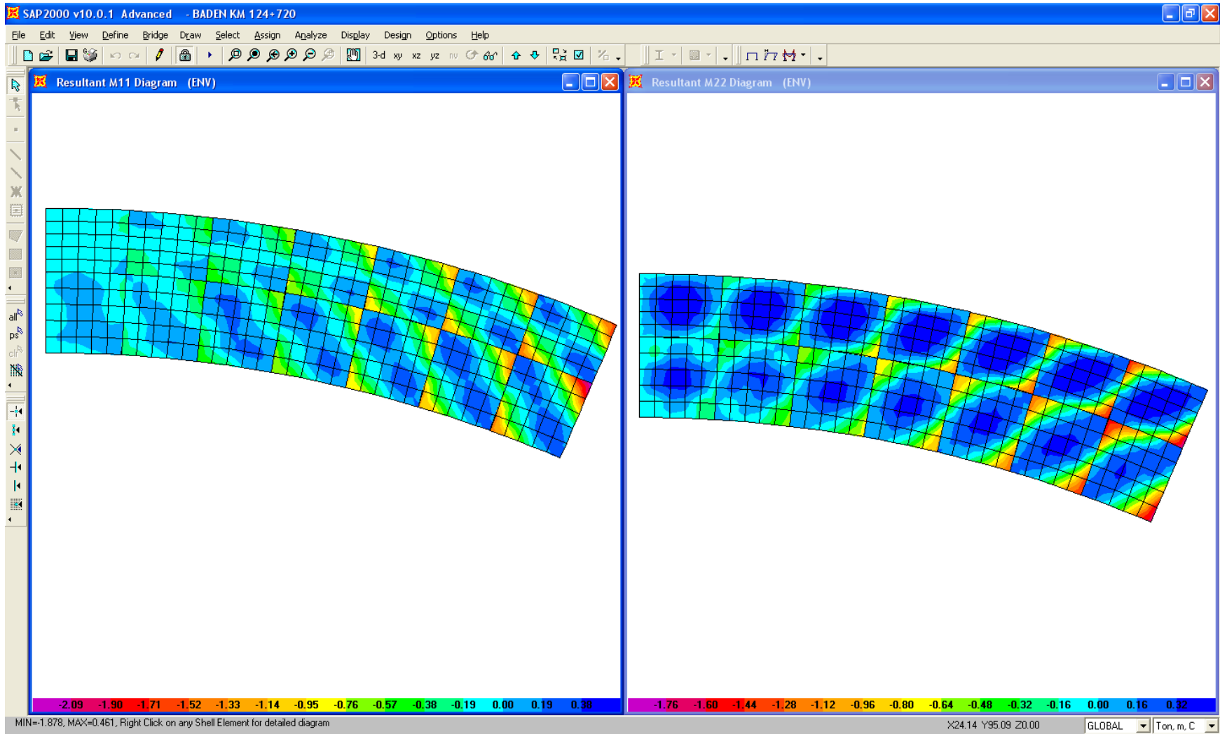
MOMENTOS MIN.EN DIRECCIONES 1 Y 2
