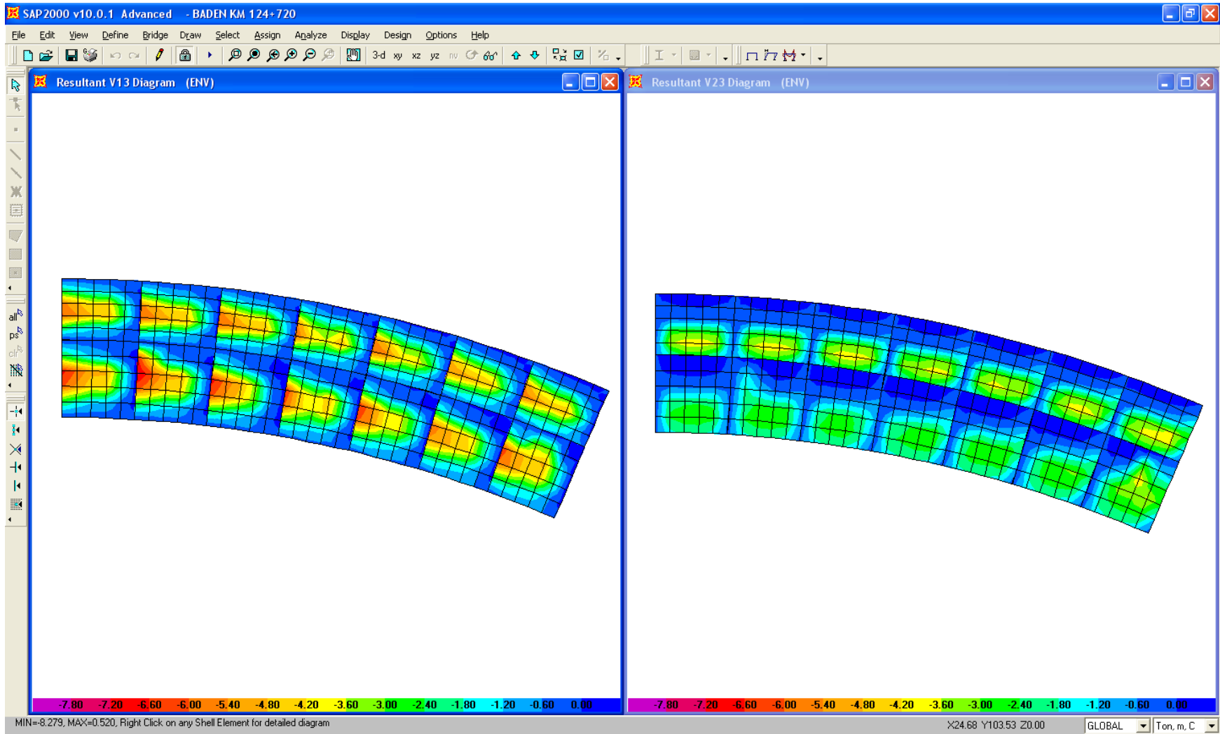
CORTANTES MIN.EN DIRECCIONES 1 Y 2
