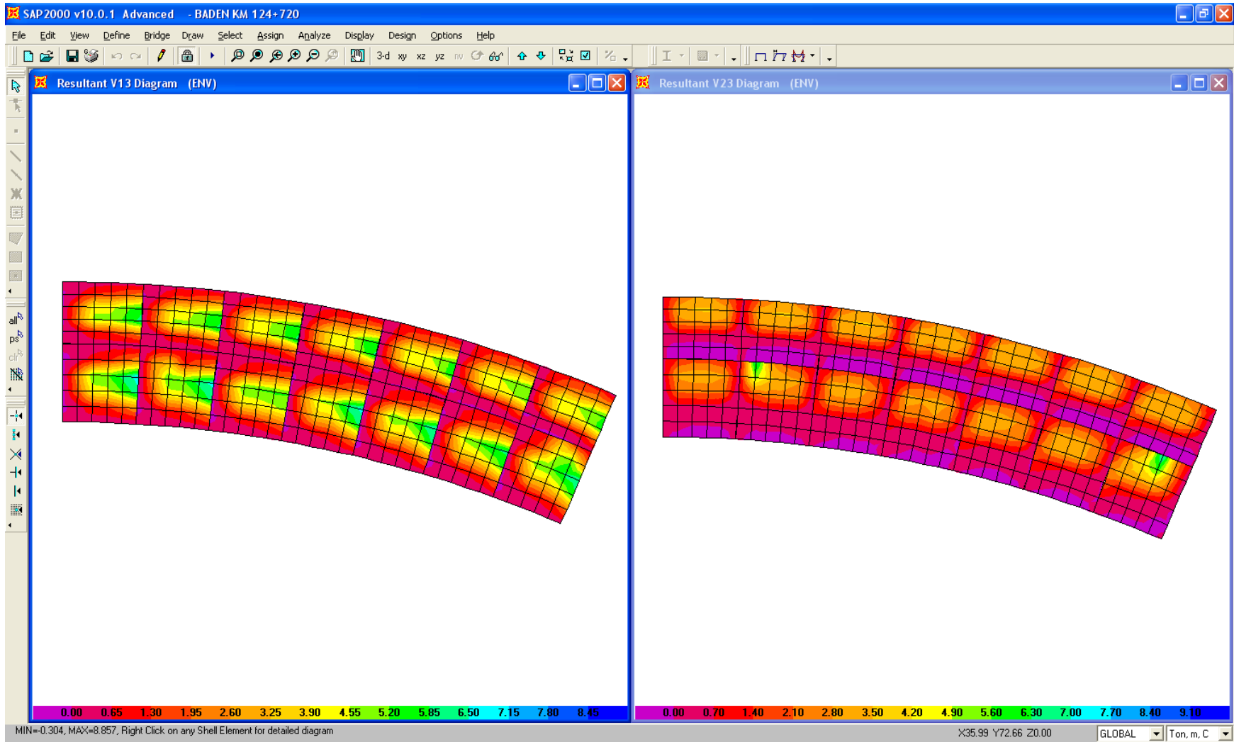
CORTANTES MAX.EN DIRECCIONES 1 Y 2
