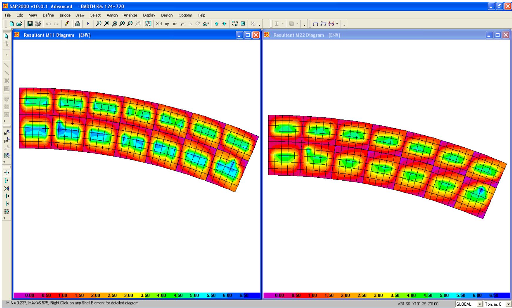
MOMENTOS MAX.EN DIRECCIONES 1 Y 2
