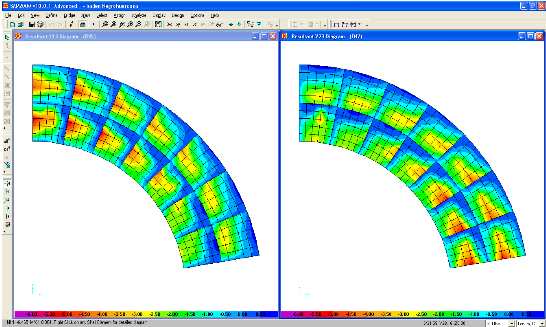
CORTANTES MIN. EN LAS DIRECCIONES 1 Y 2
