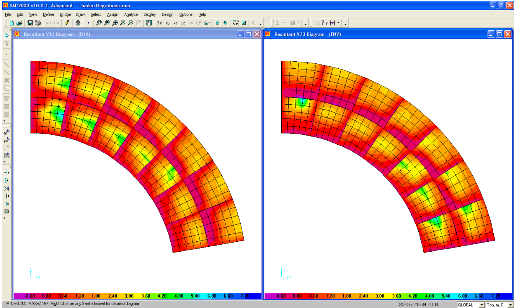
CORTANTES MAX. EN LAS DIRECCIONES 1 Y 2
