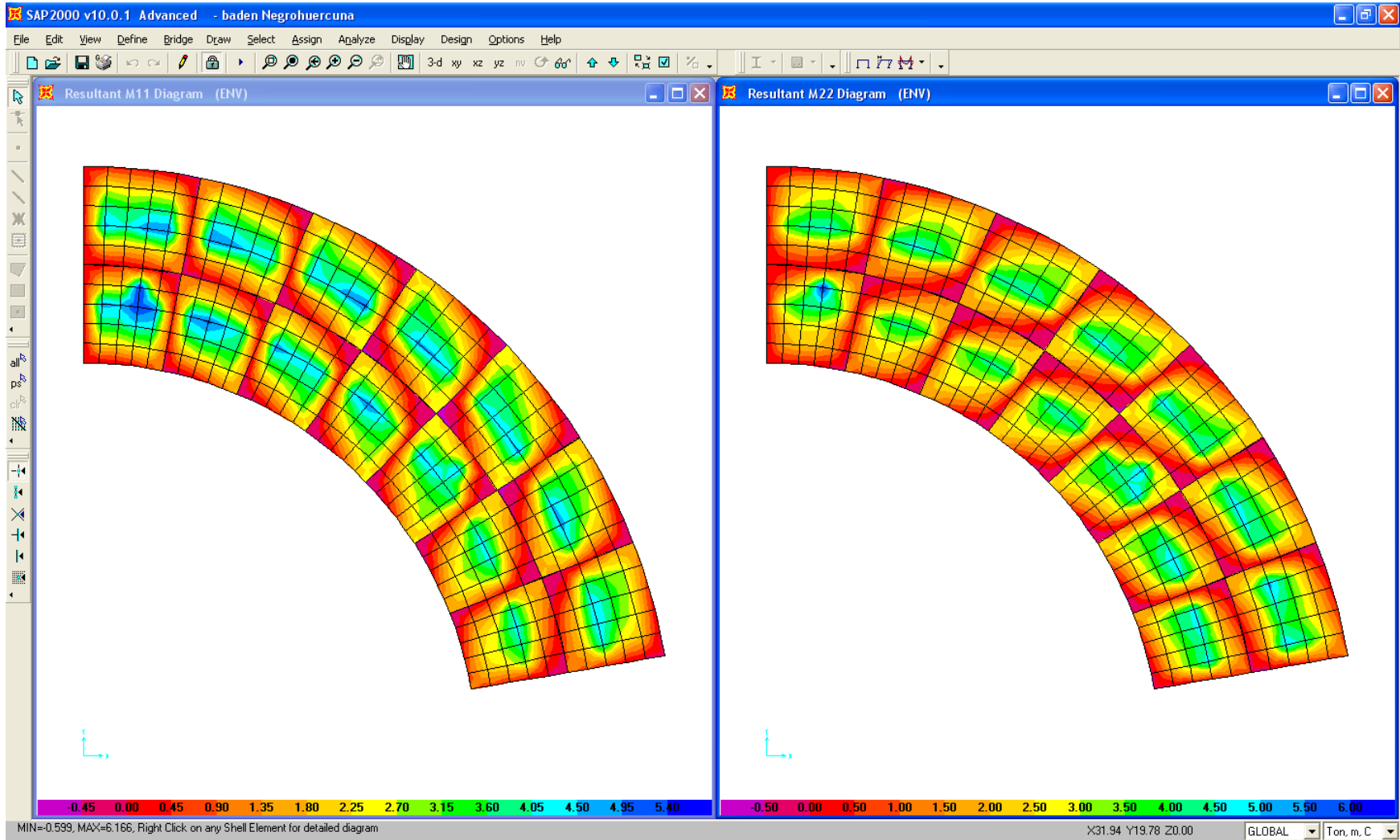
MOMENTOS MAX. EN LAS DIRECCIONES 1 Y 2
