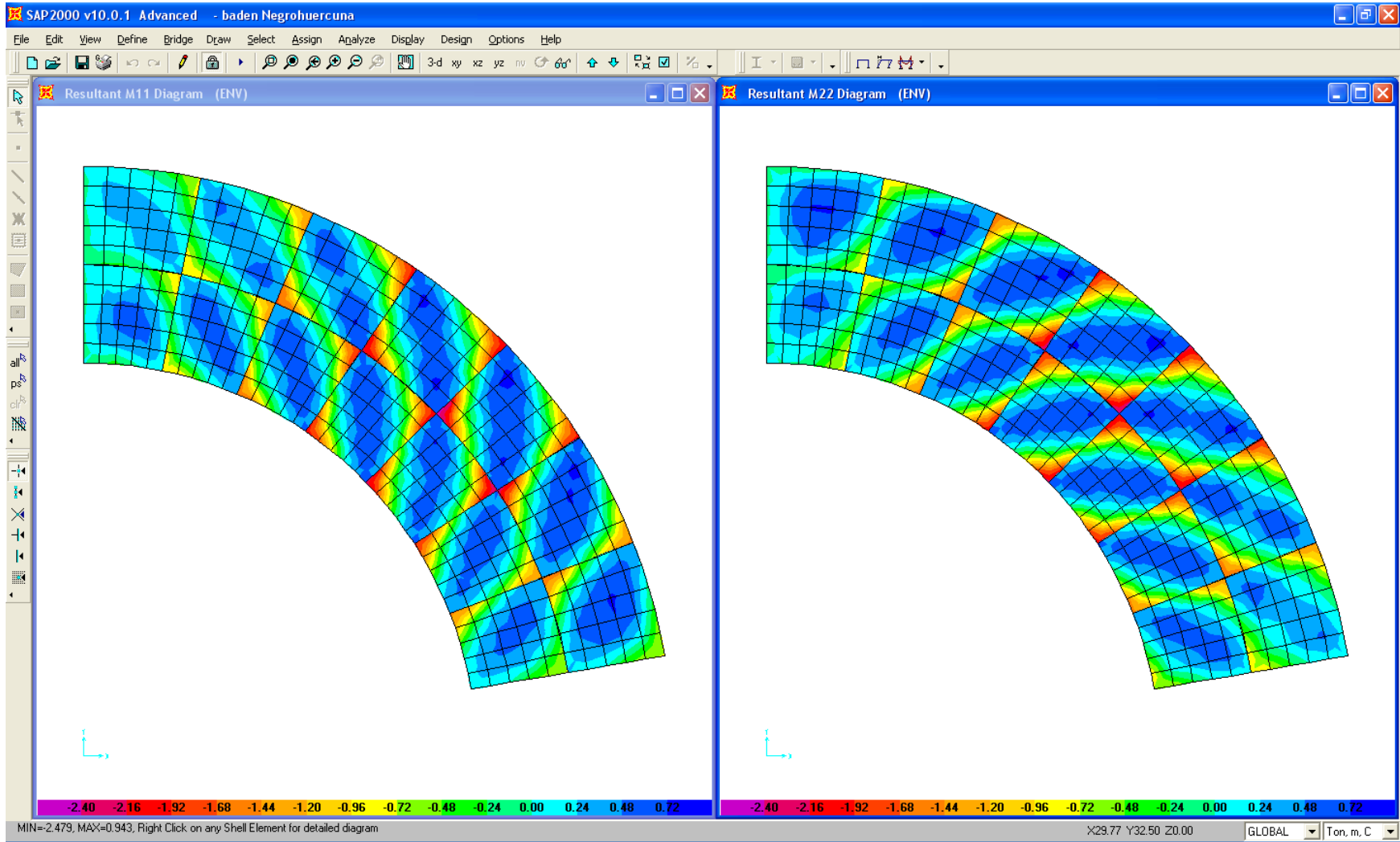
MOMENTOS MIN. EN LAS DIRECCIONES 1 Y 2
