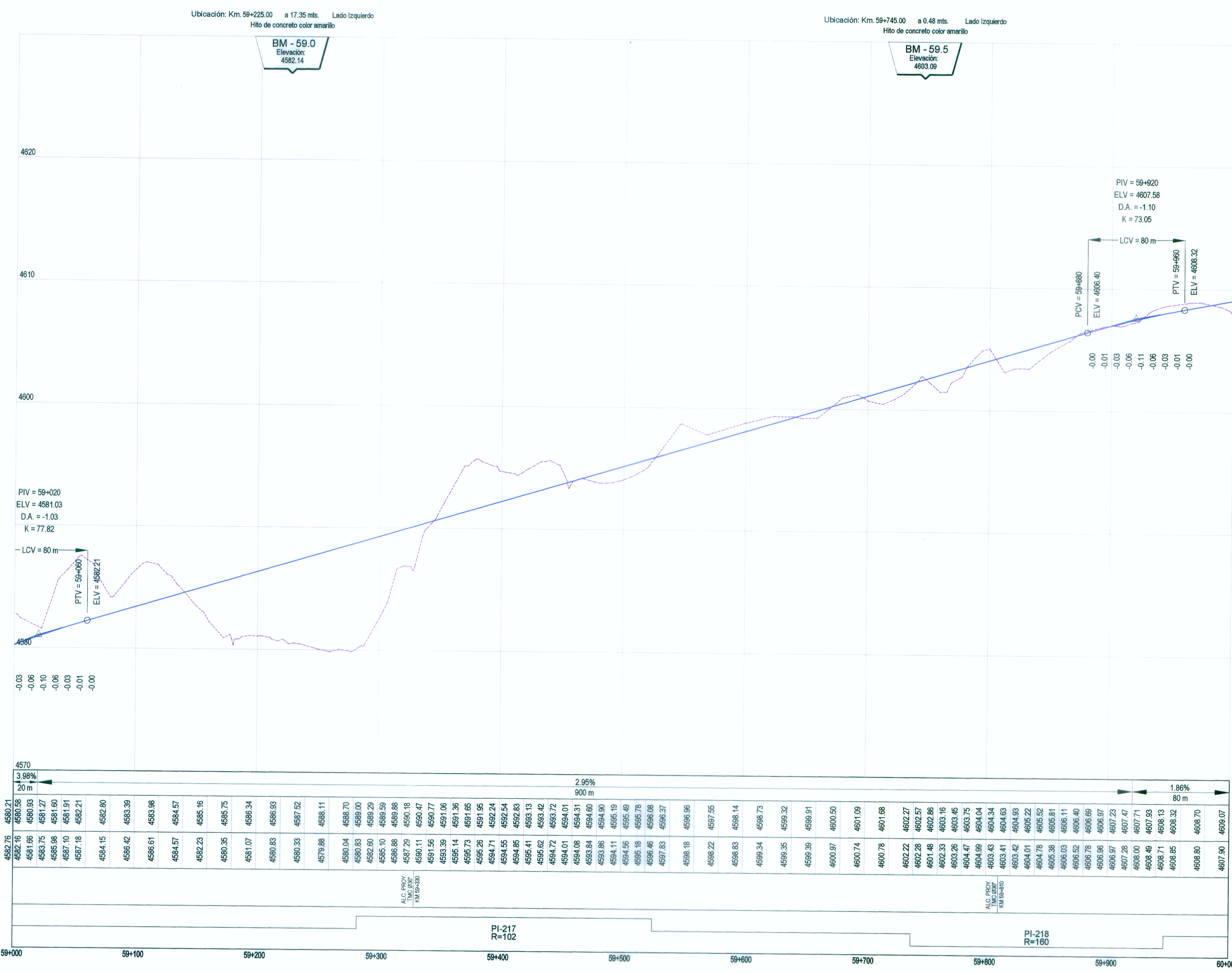
PERFIL LONGITUDINAL H: 1/2,000 V: 1/200
