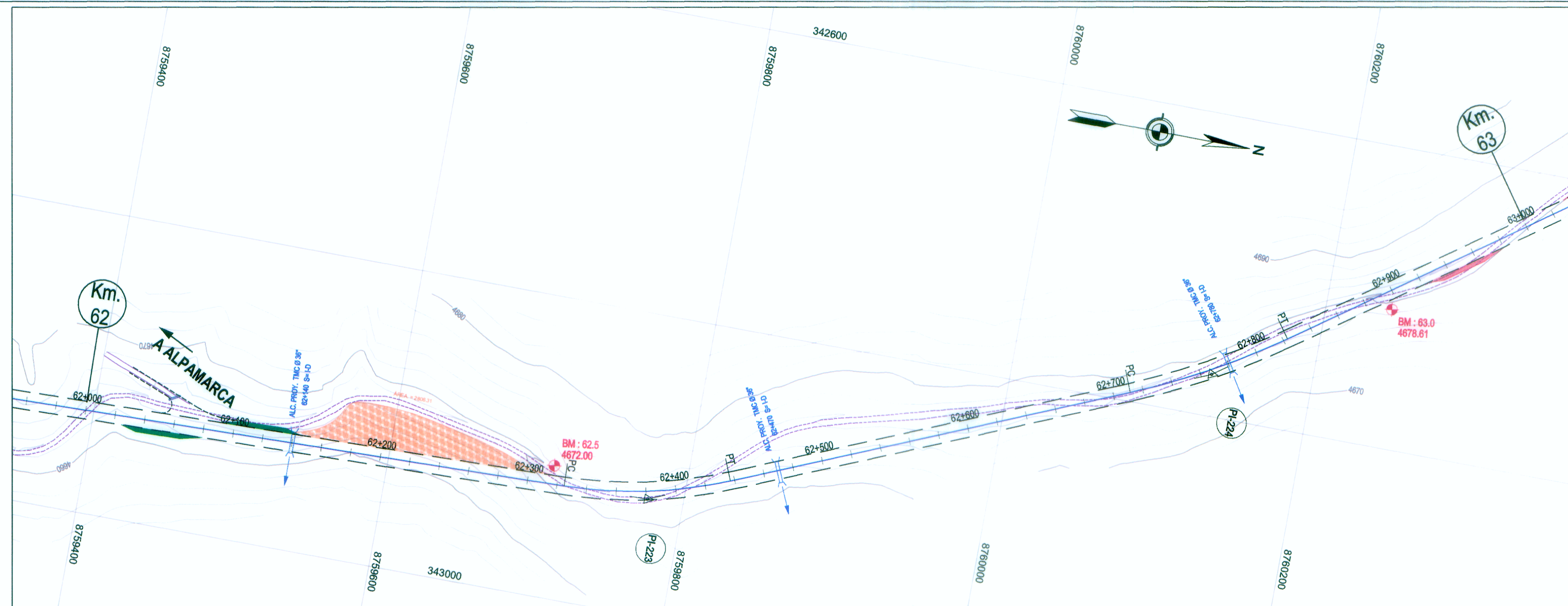
PLANTA
