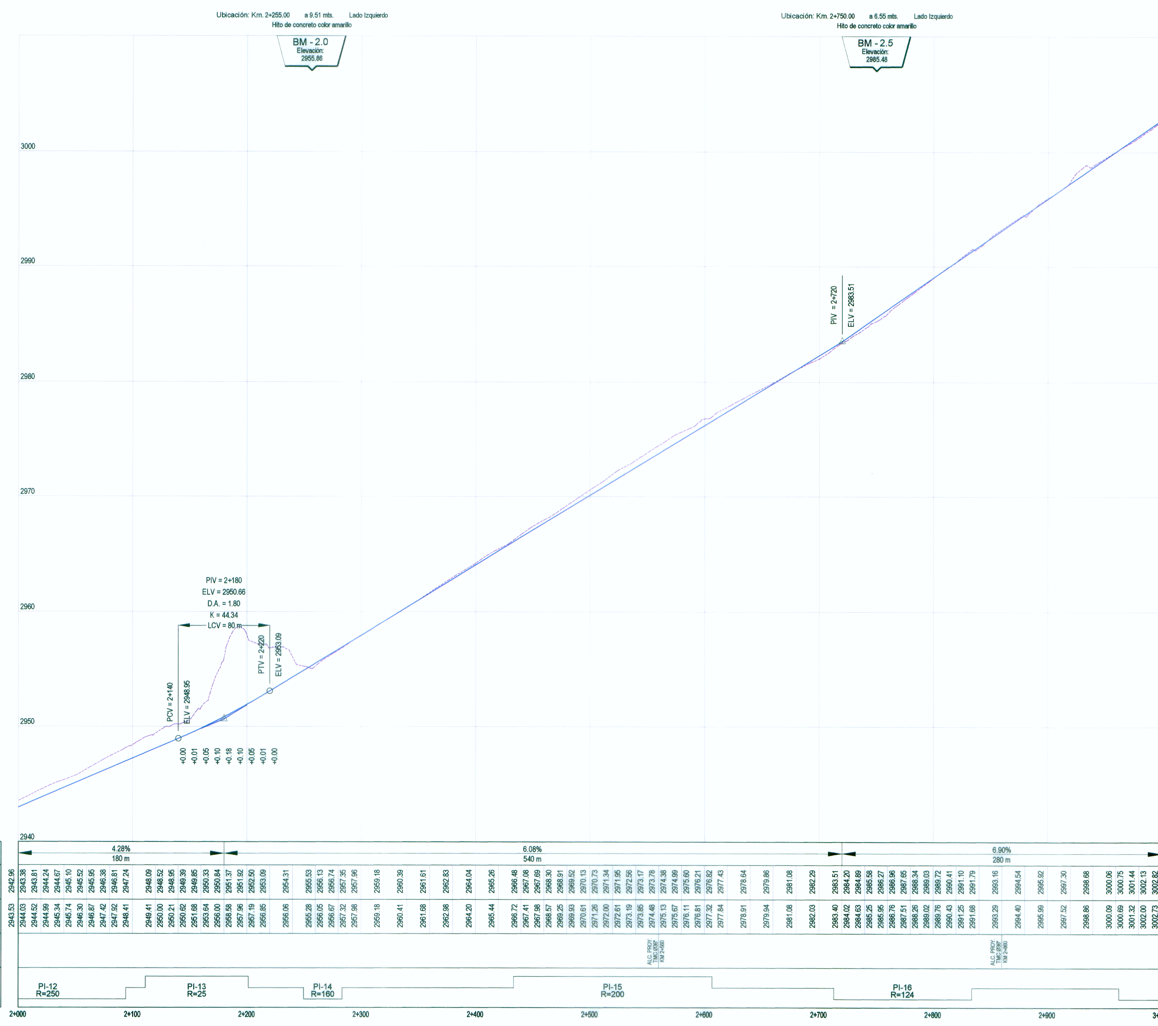
PERFIL LONGITUDINAL H: 1/2,000 V: 1/200
