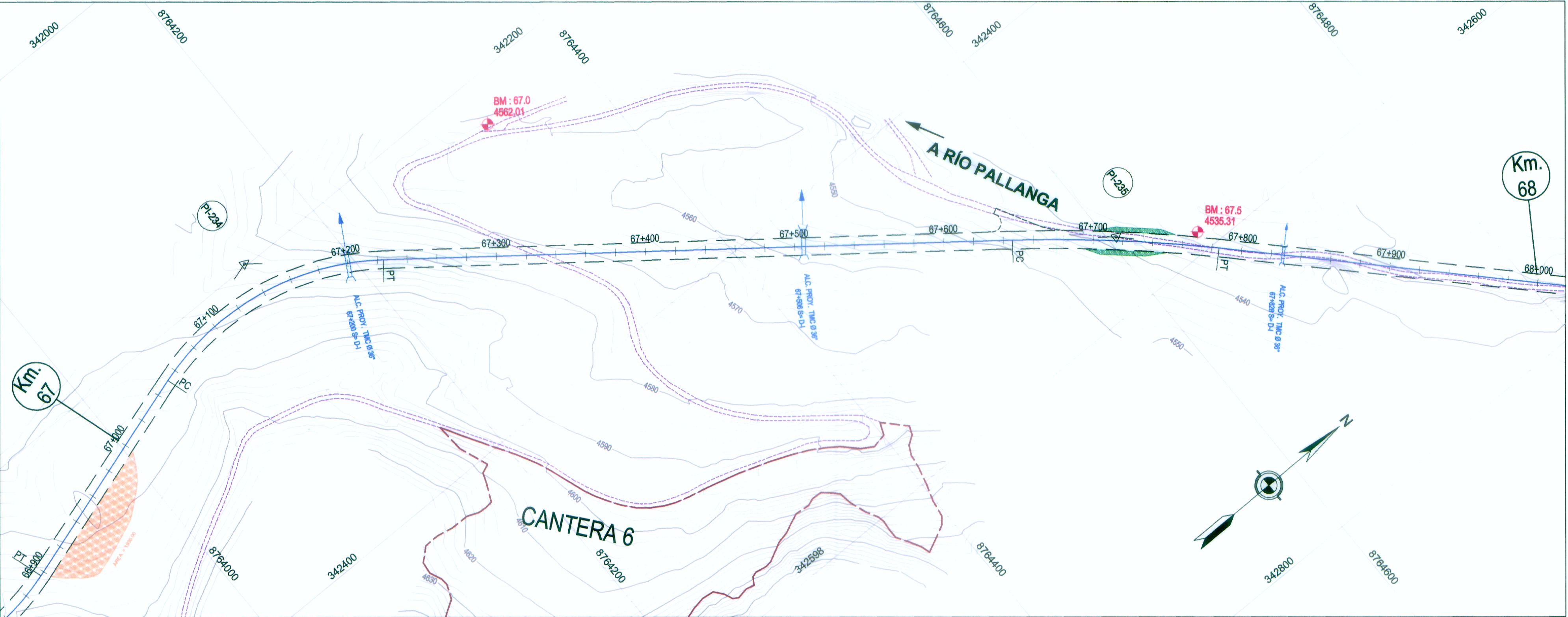
PLANTA H: 1/2,000
