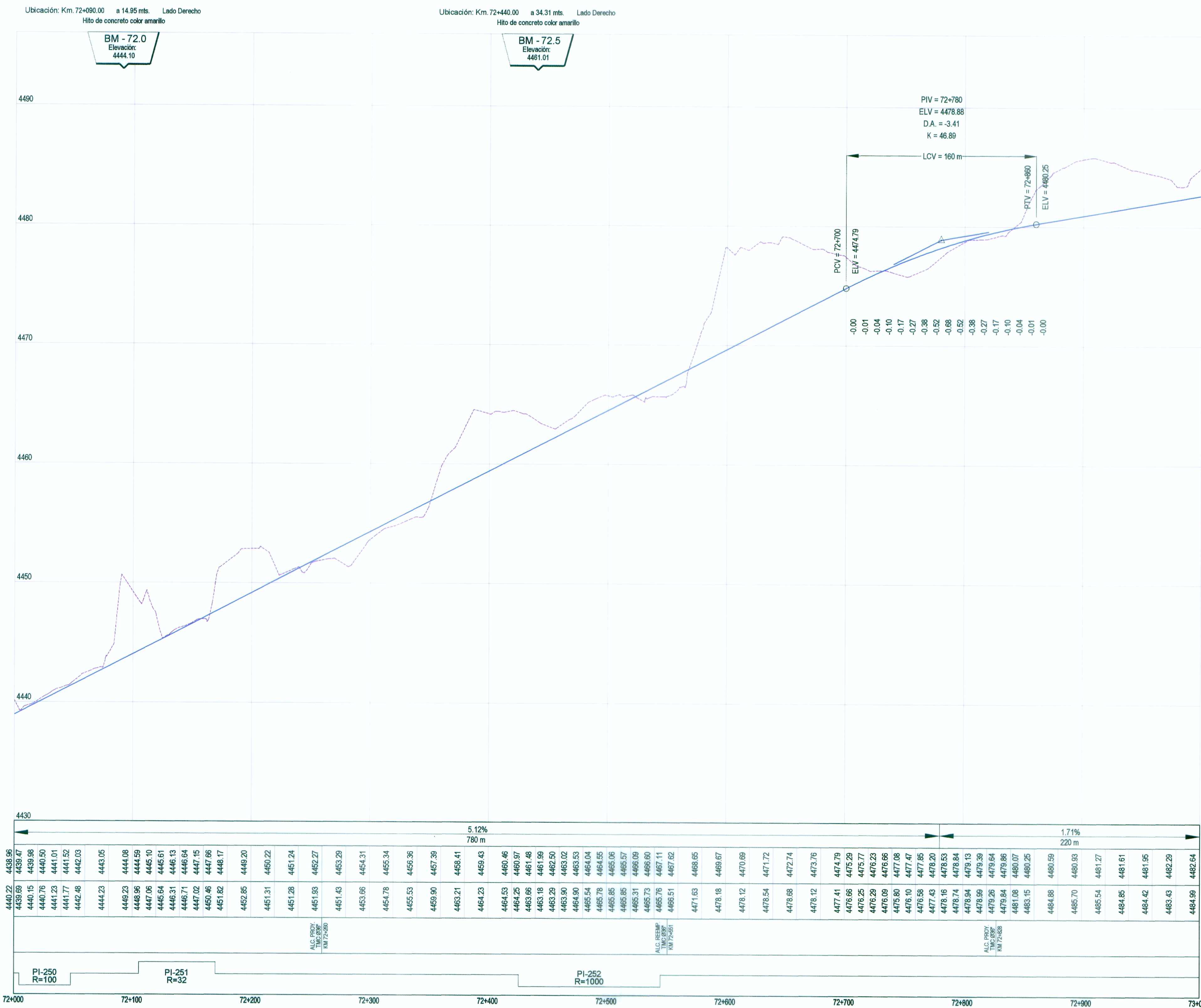
PERFIL LONGITUDINAL H: 1/2,000 V: 1/200
