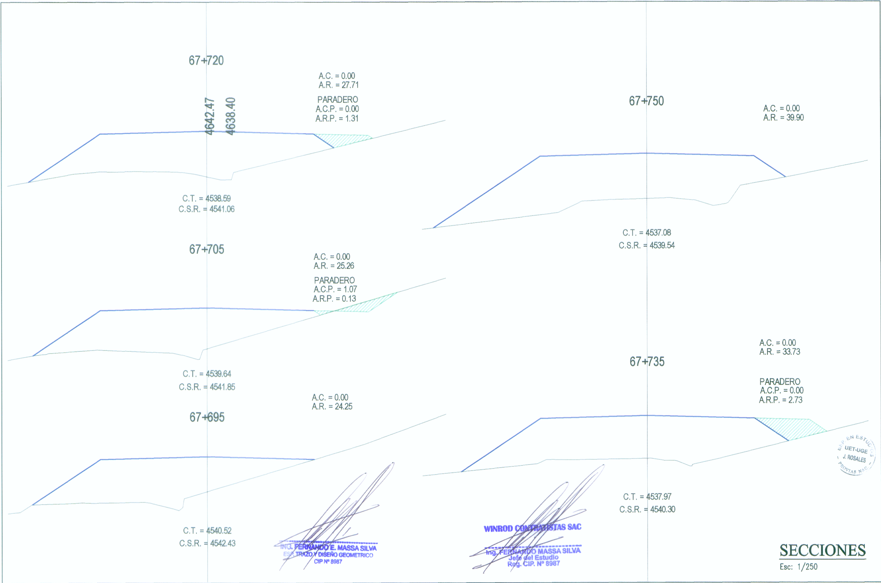
SECCIONES Esc: 1/250
