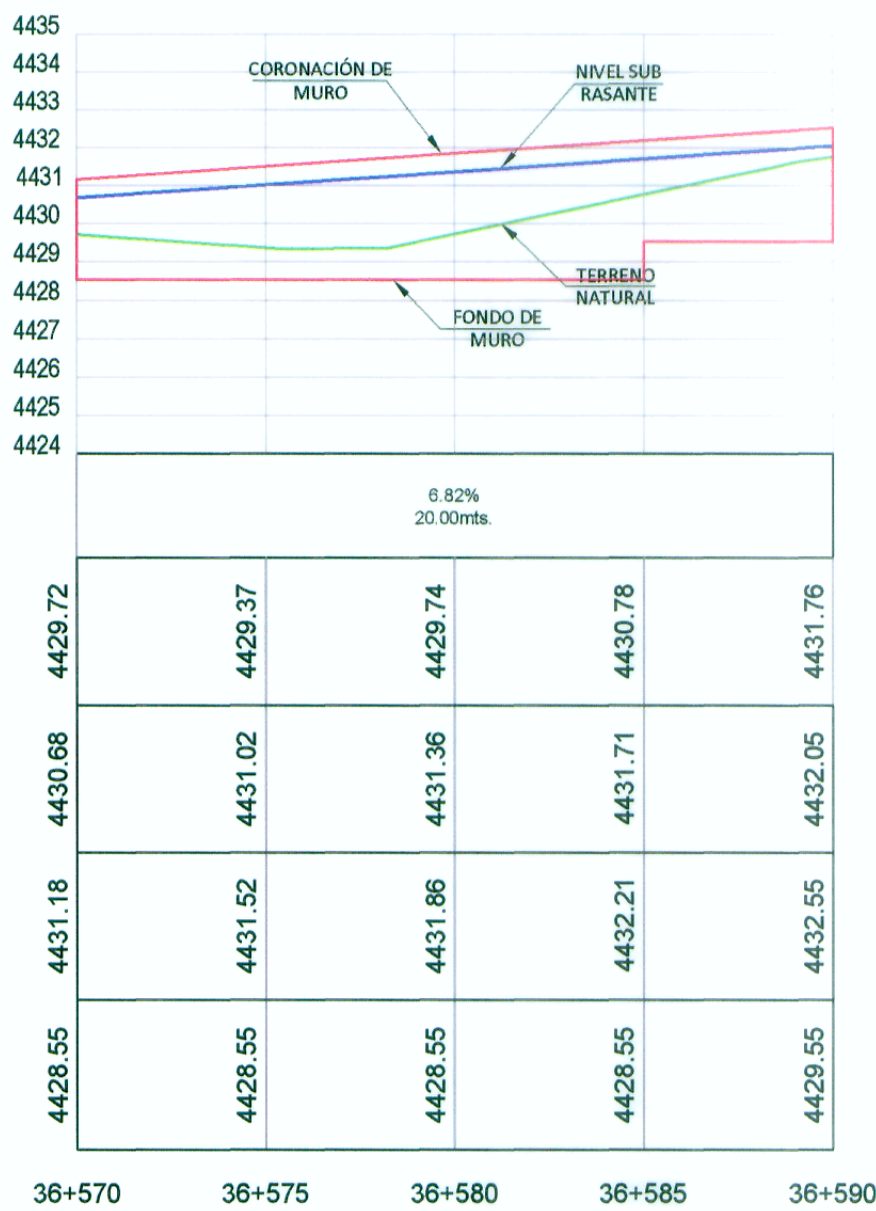
Muro 36+570 - 36+590
