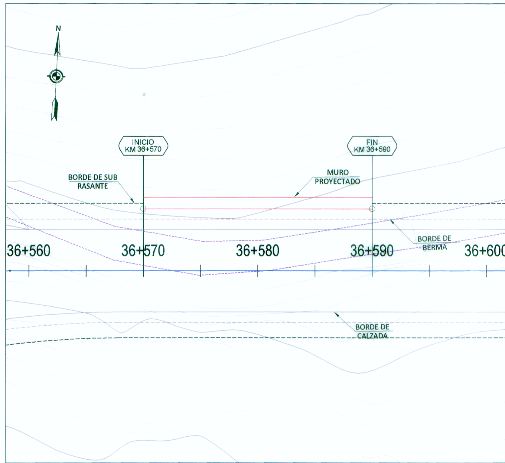
PLANTA
