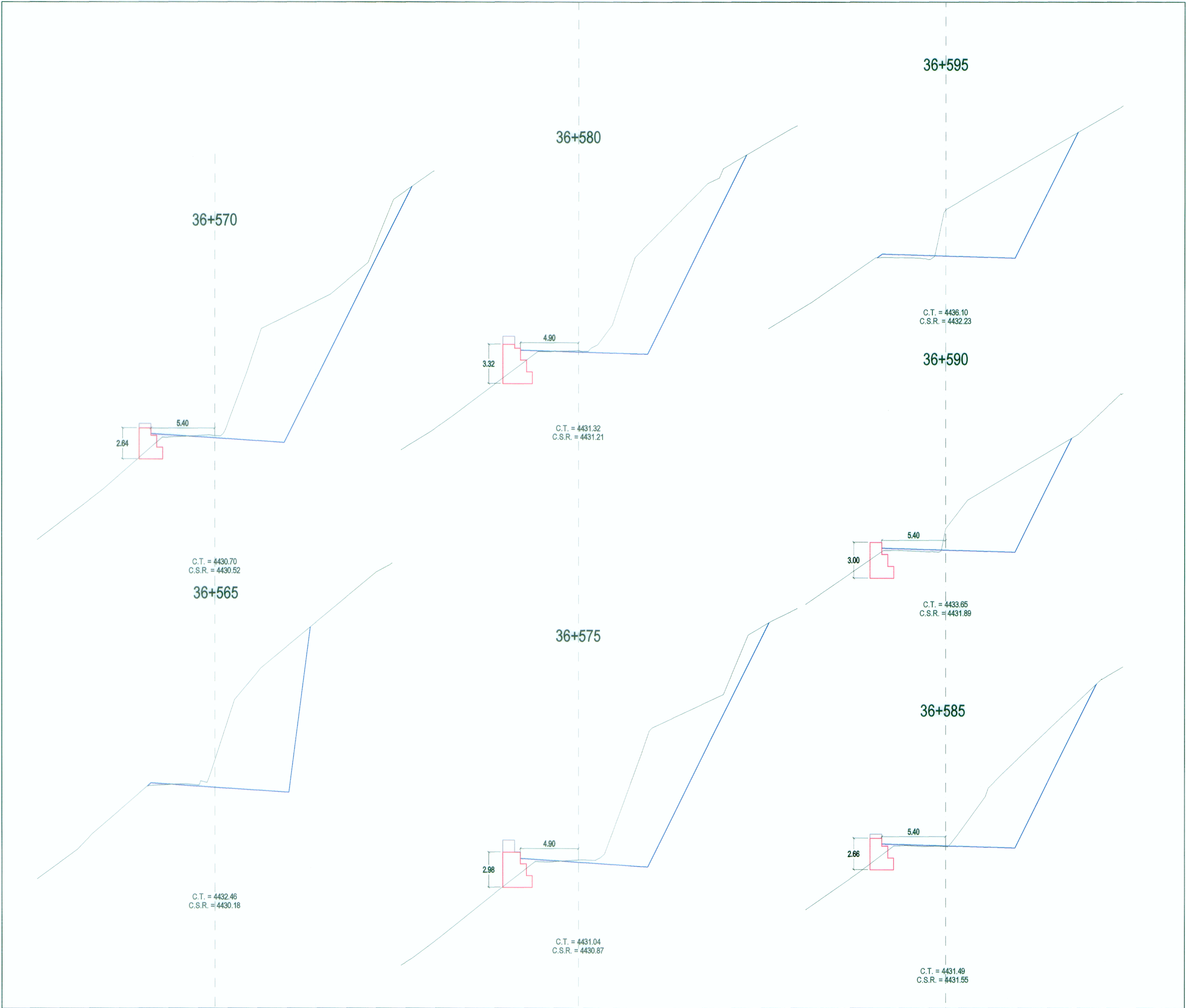
SECCIONES TRANSVERSALES
