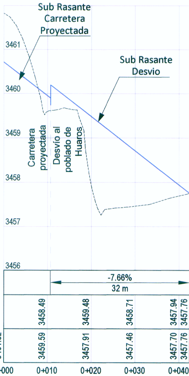
PERFIL LONGITUDINAL ESC: 1/500
