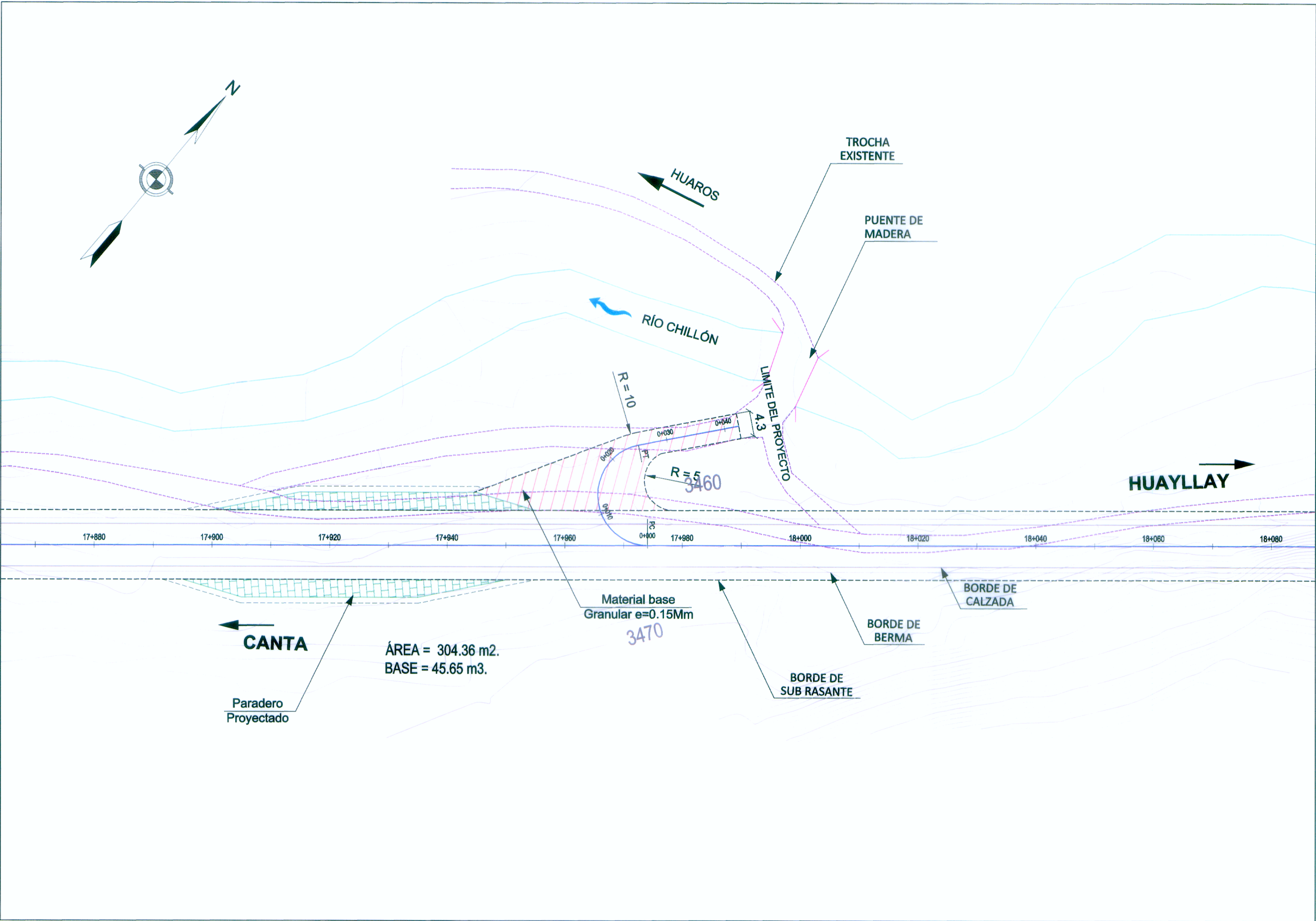
PLANTA ESC: 1/500
