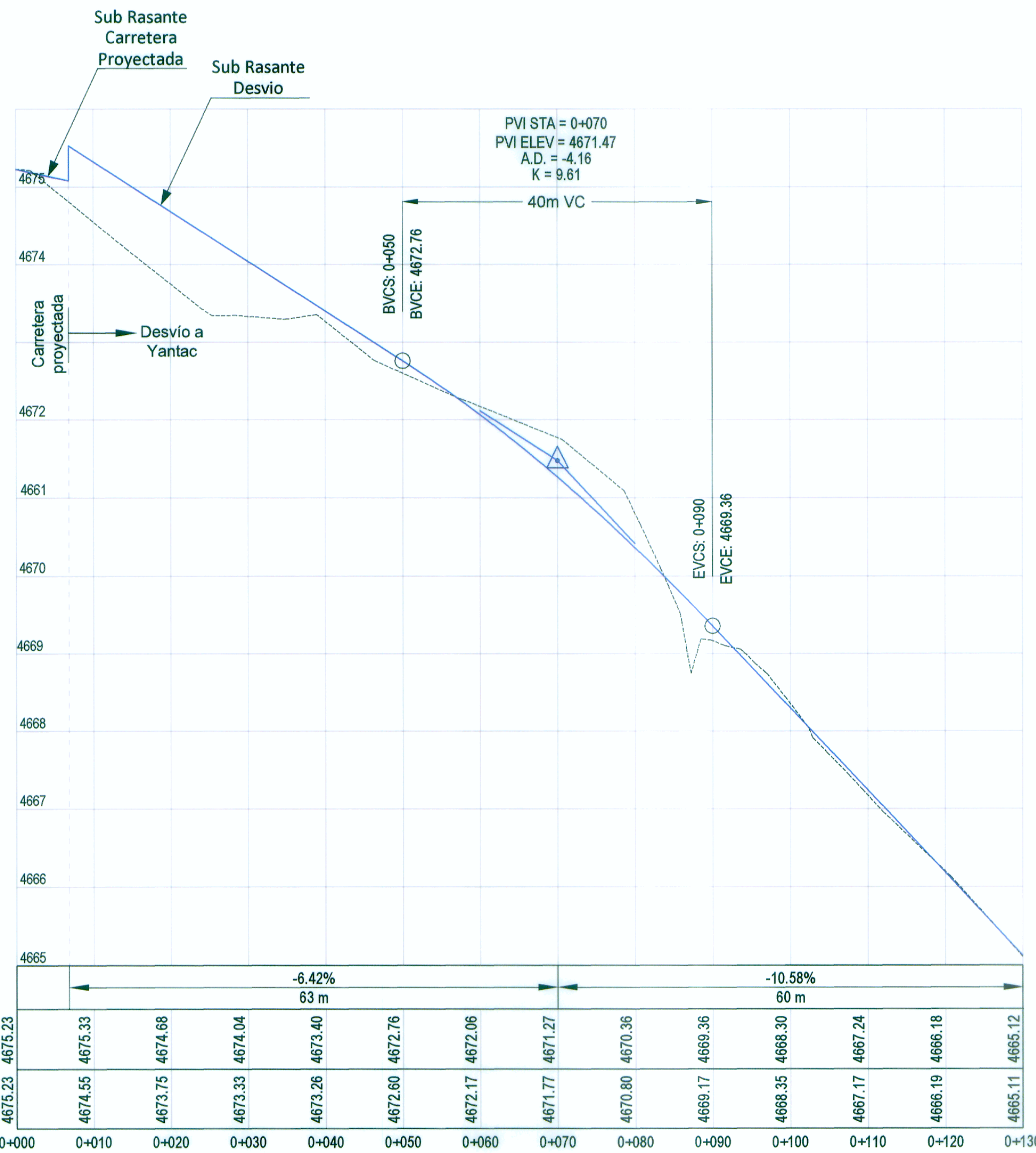
PERFIL LONGITUDINAL ESC: 1/500
