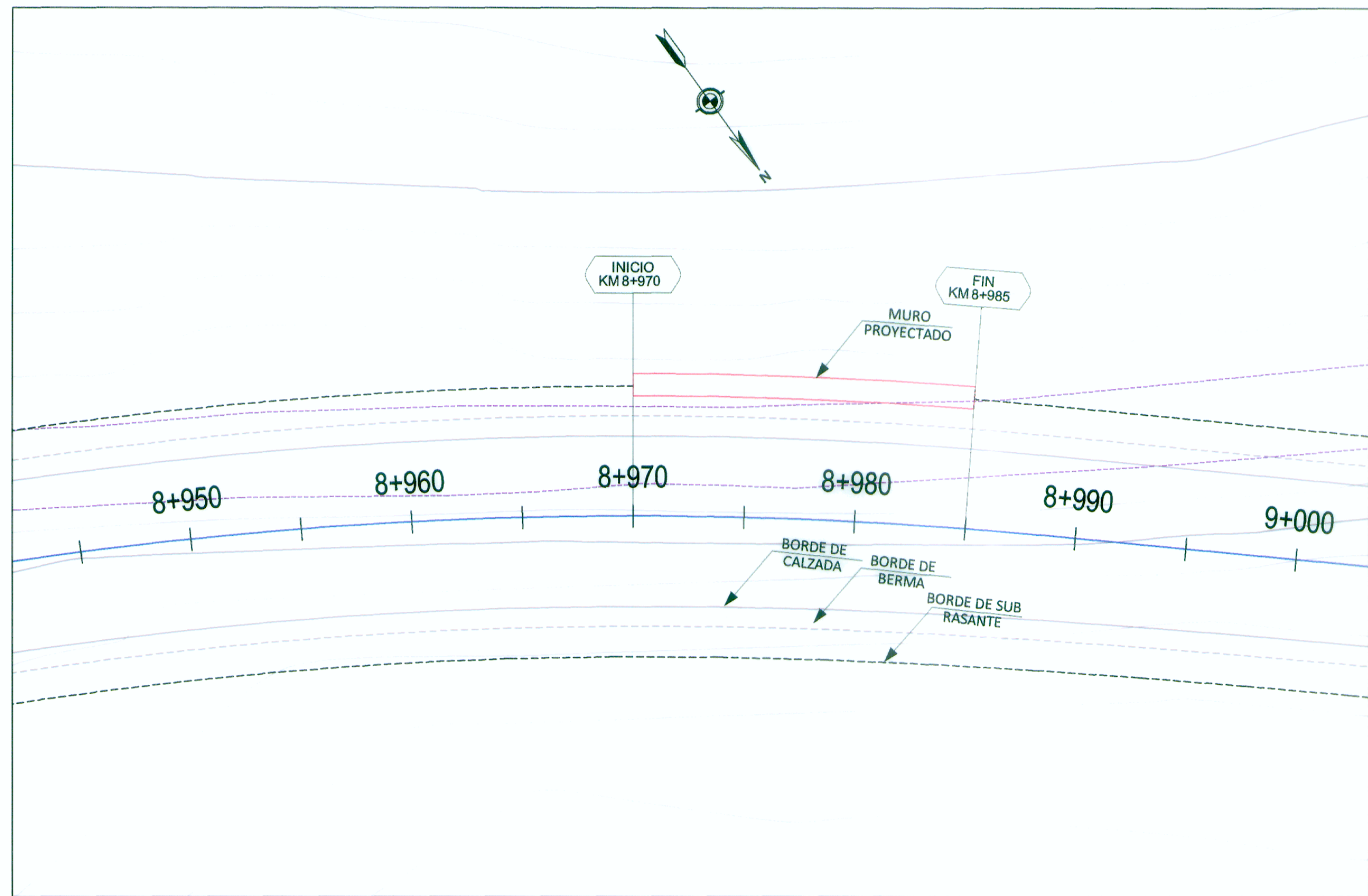
PLANTA
