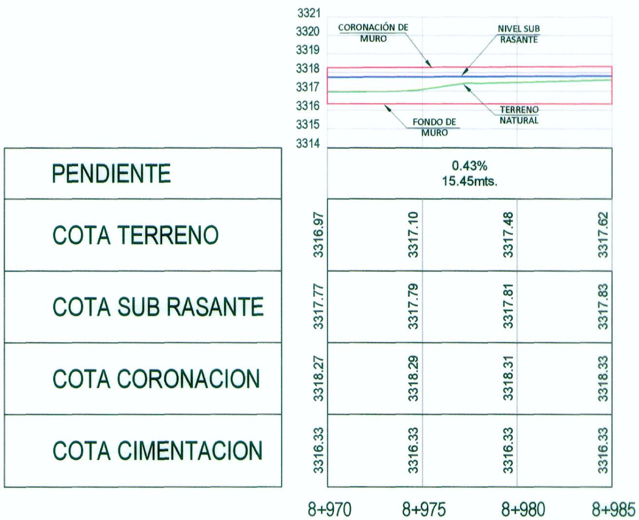
PERFIL LONGITUDINAL
