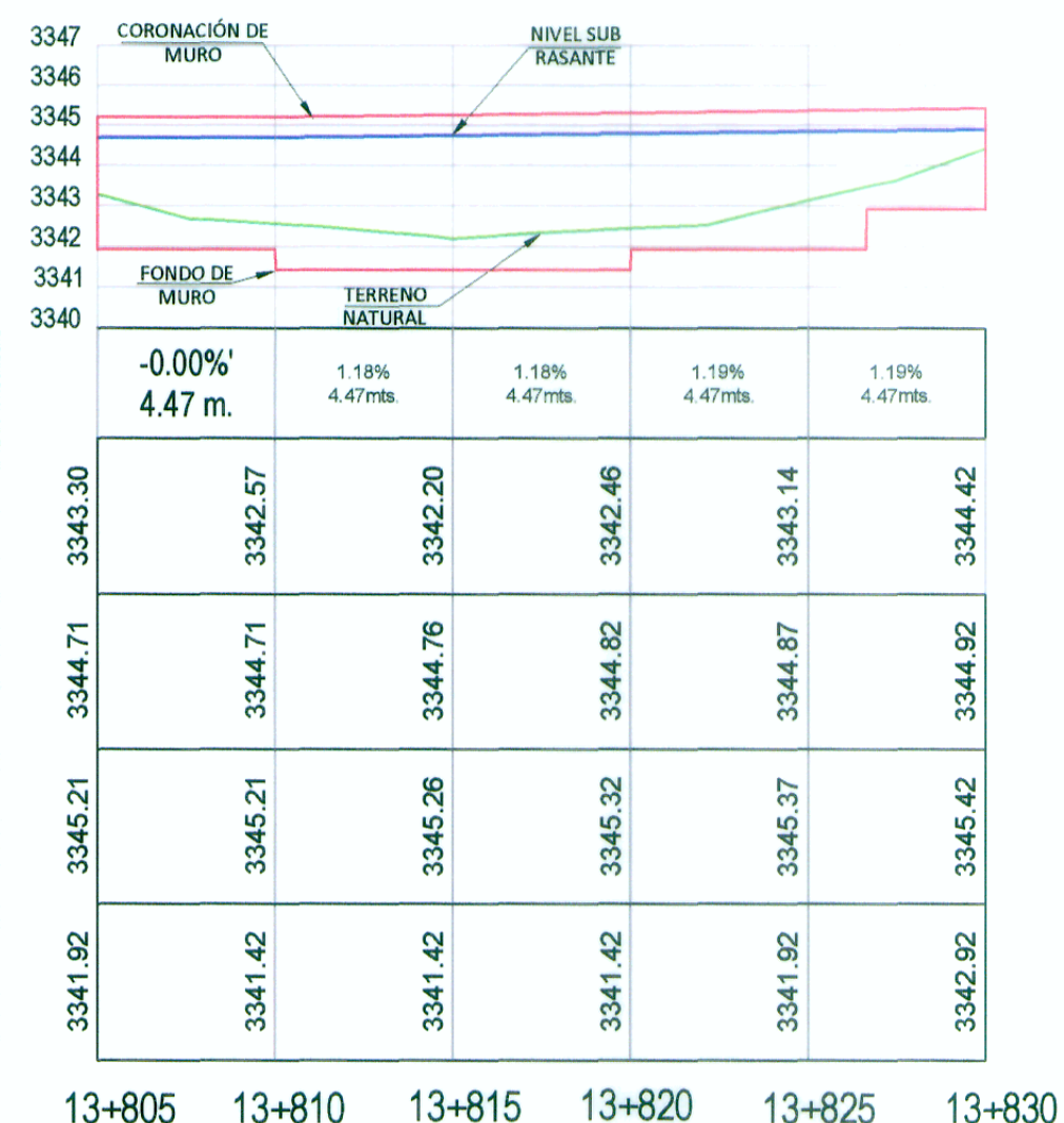
PERFIL LONGITUDINAL
