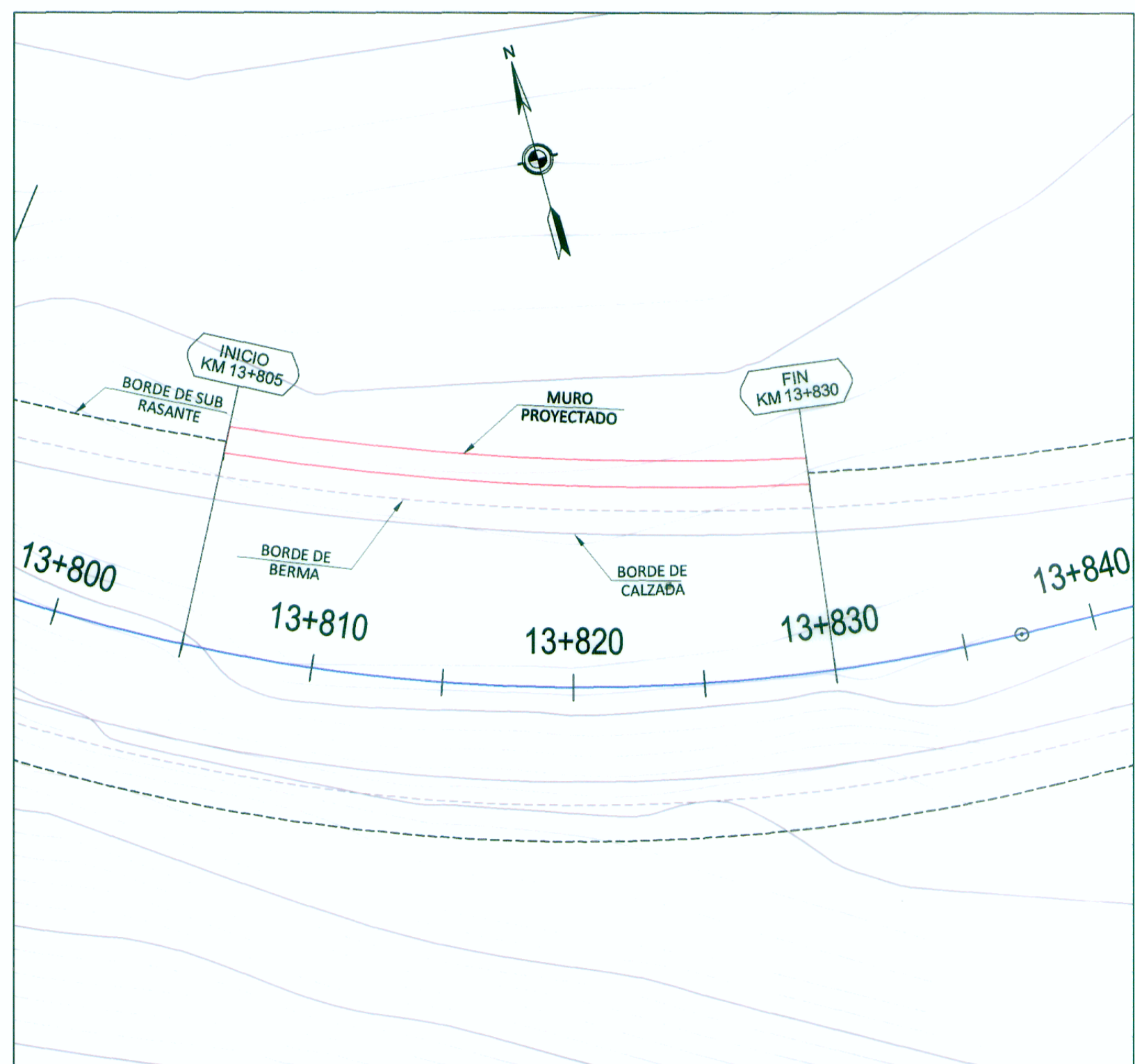
PLANTA
