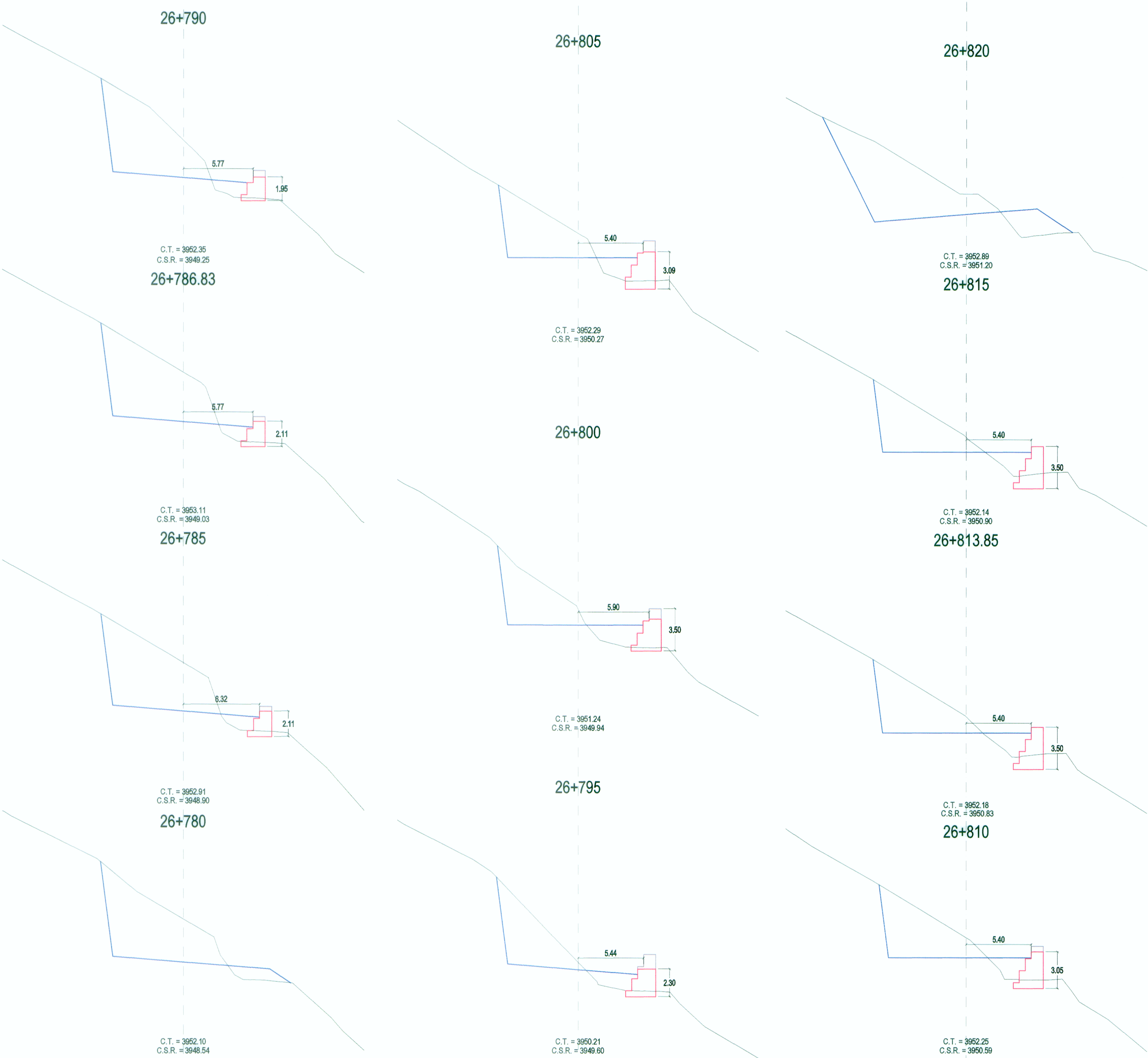
SECCIONES TRANSVERSALES
