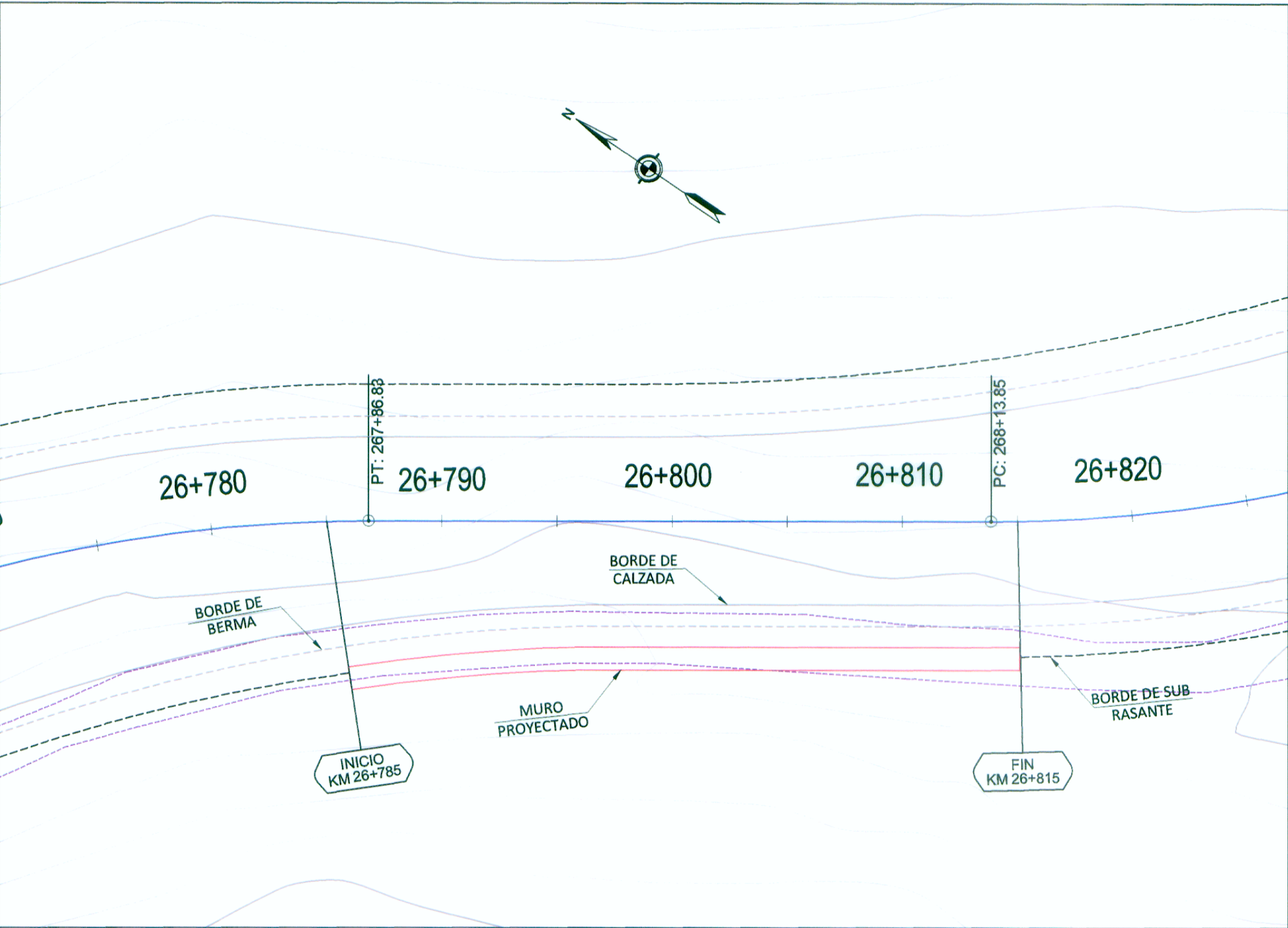
PLANTA
