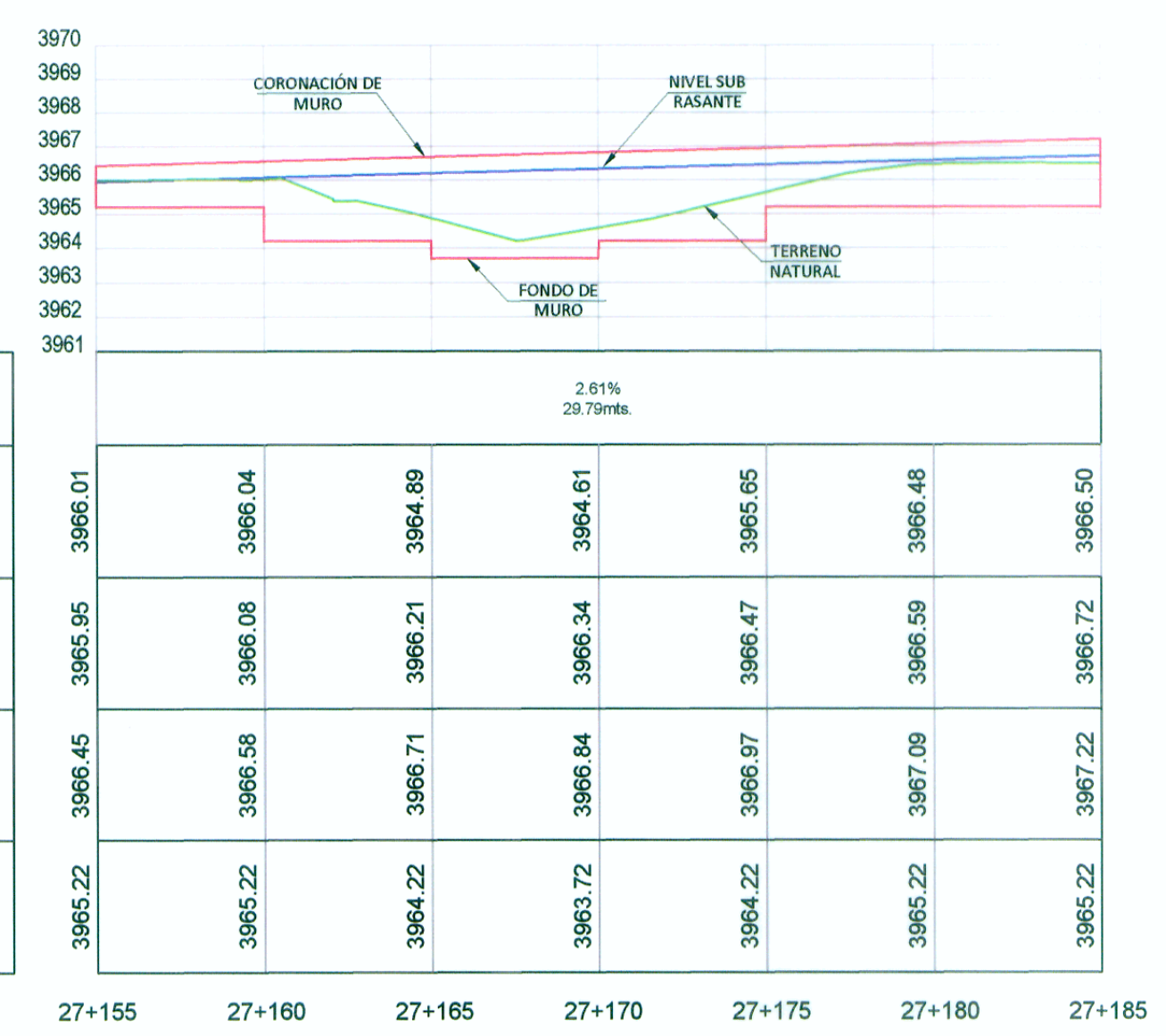
PERFIL LONGITUDINAL
