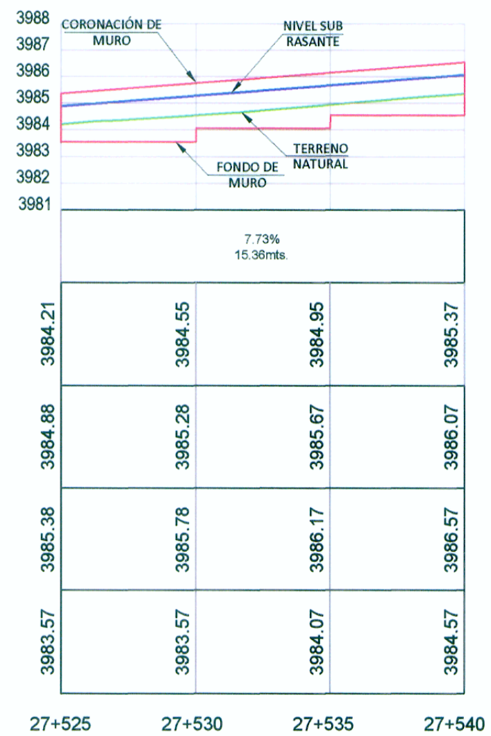
PERFIL LONGITUDINAL
