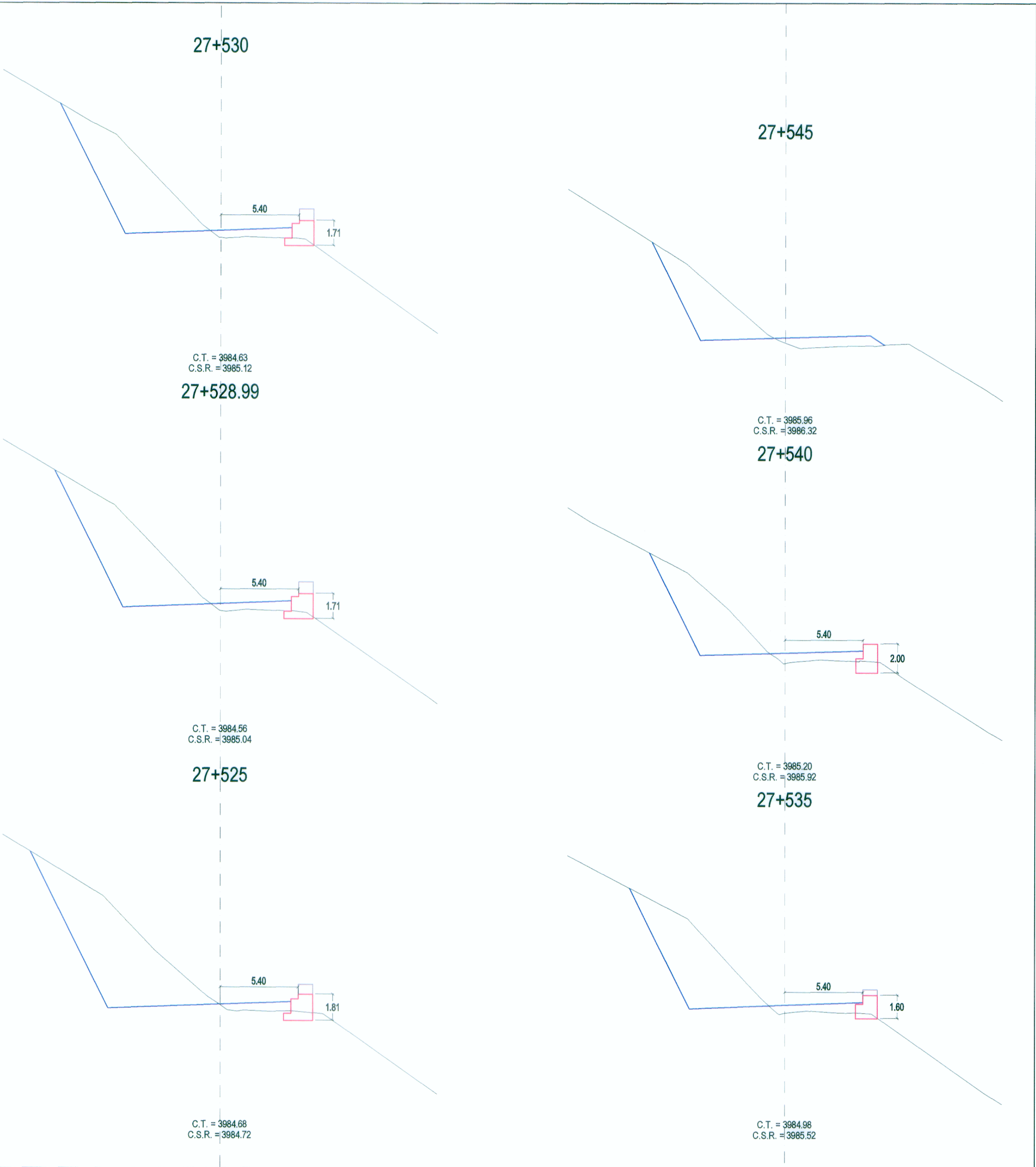
SECCIONES TRANSVERSALES
