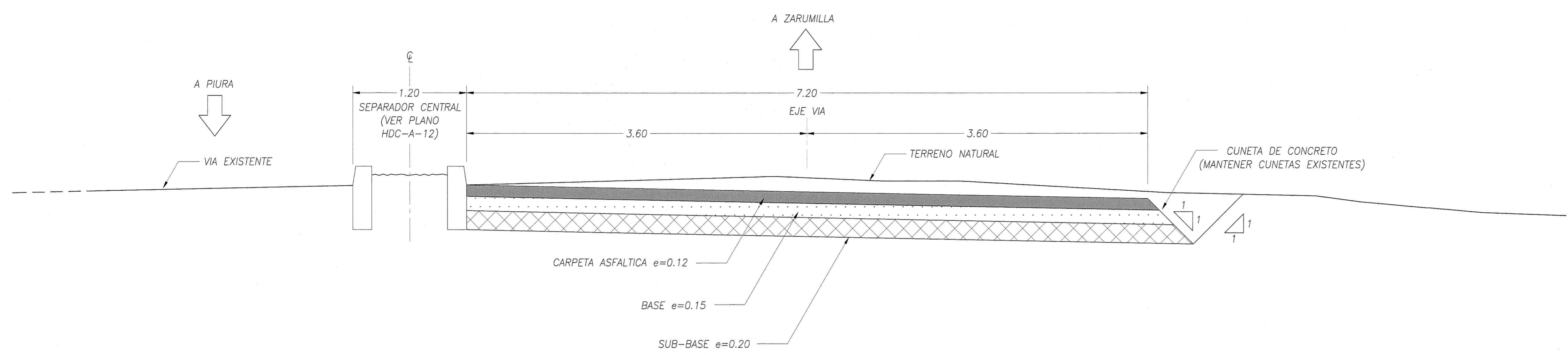
SECCION TRANSVERSAL TIPICA EN CORTE ESC: 1/50
