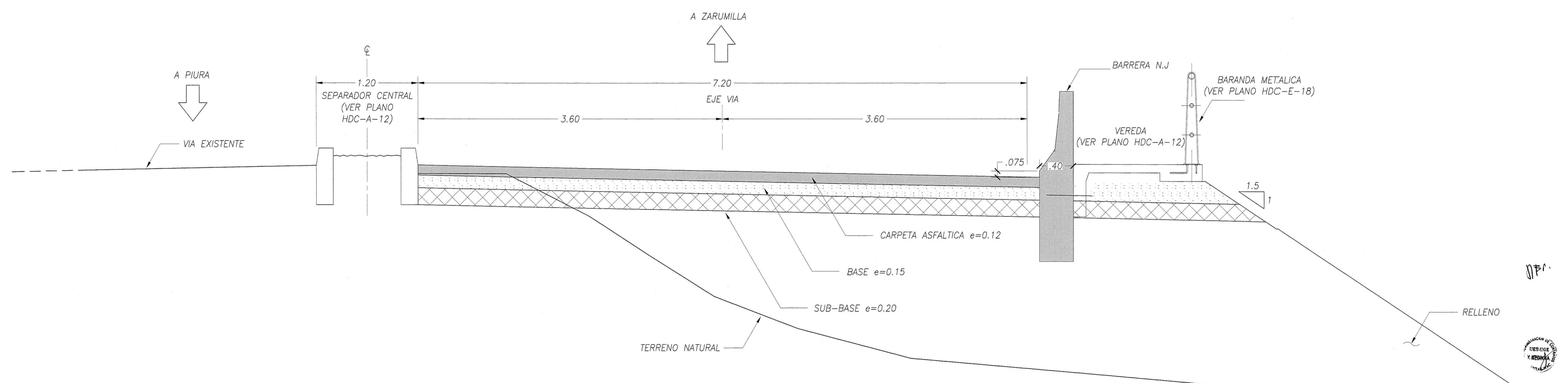
SECCION TRANSVERSAL TIPICA EN RELLENO ESC: 1/50
