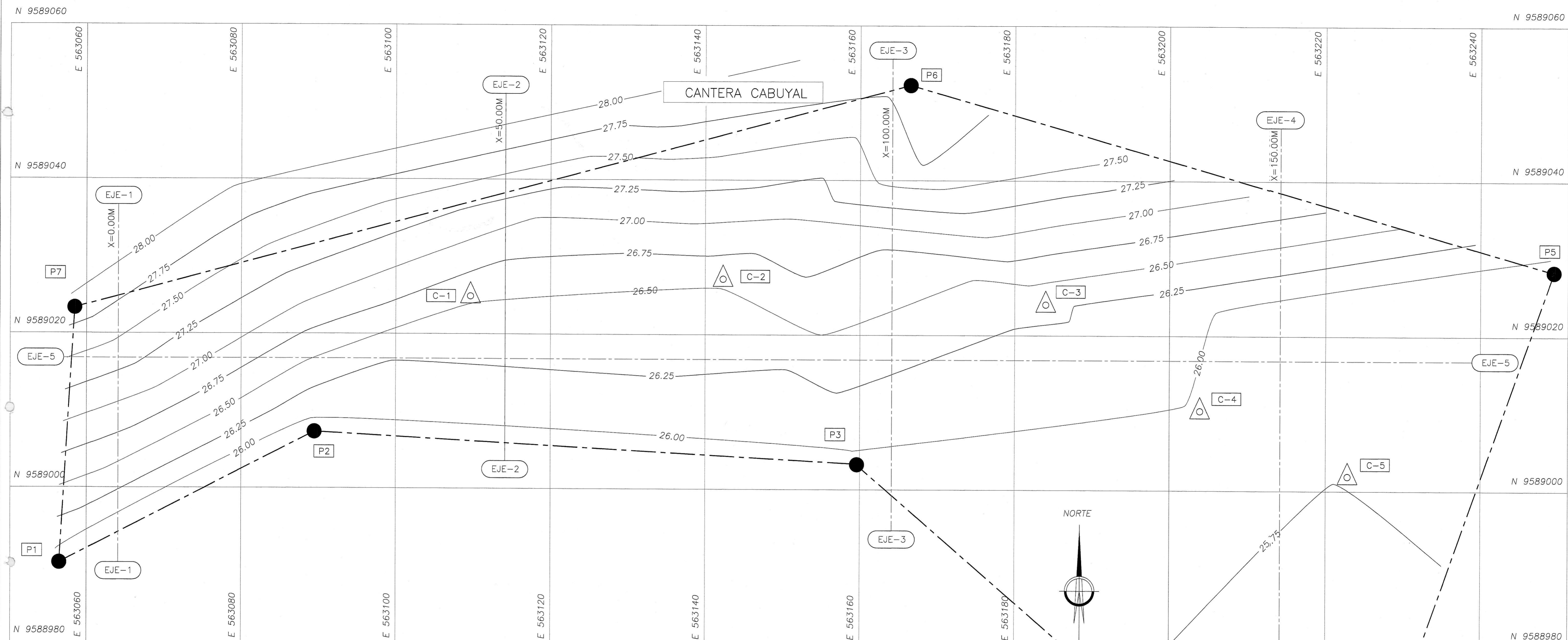
TOPOGRAFIA CANTERA CABUYAL ESC:1/500
