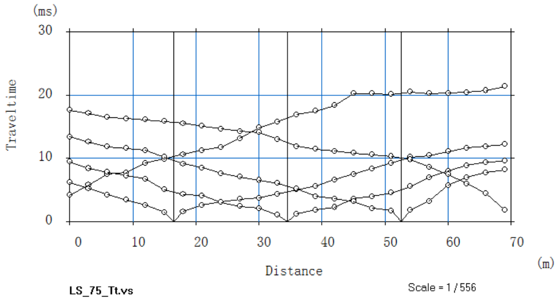
Imagen 75: Dromocrona LS 75
