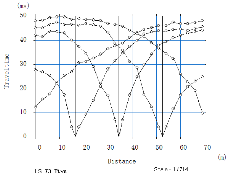
Imagen 73: Dromocrona LS 73
