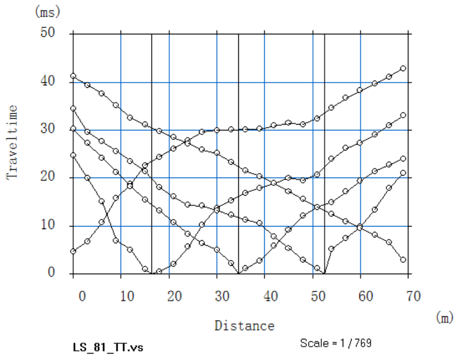
Imagen 81: Dromocrona LS 81
