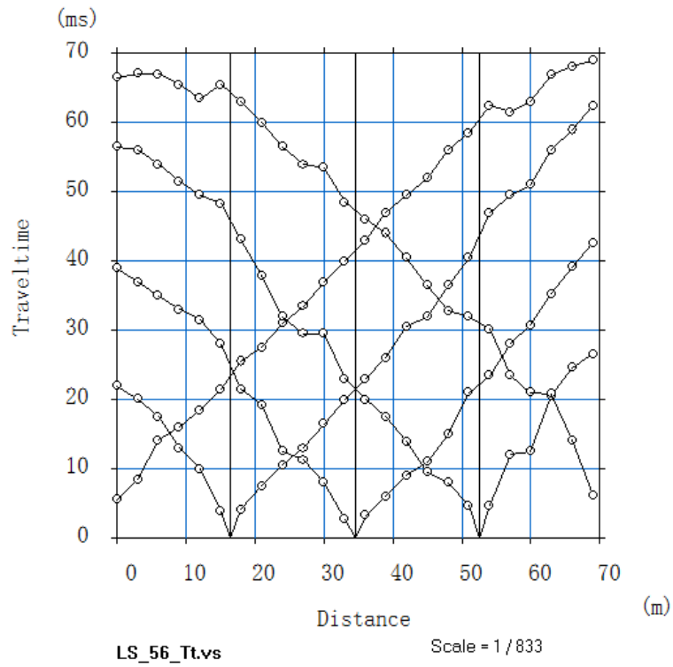
Imagen 56: Dromocrona LS 56
