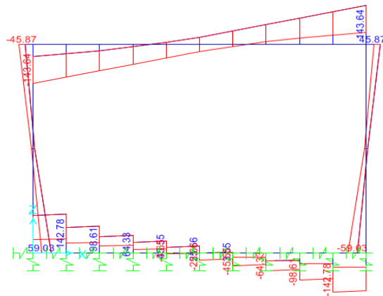
Diagrama de Fuerza Cortante
