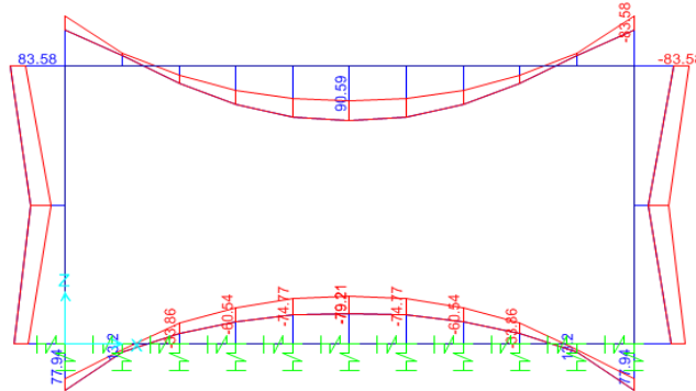
Diagrama de Momento Flector
