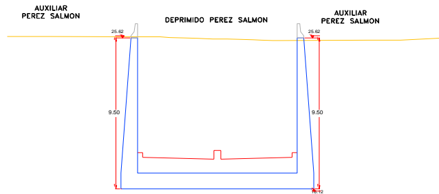
CT:25.554 CR:17.946 SECCIÓN EN RAMPA
