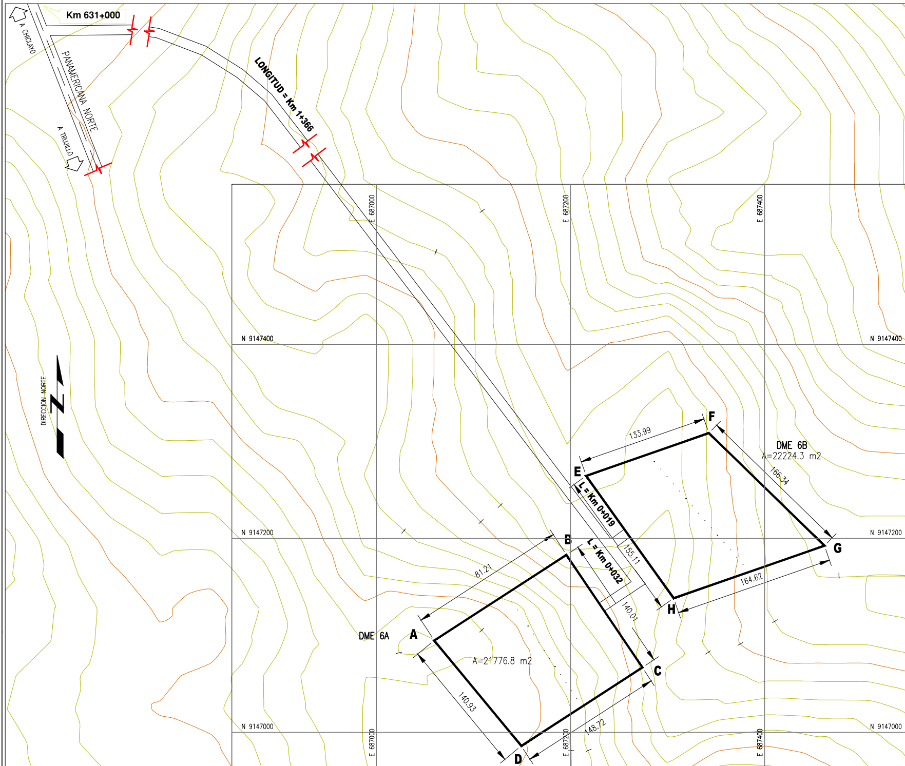
PLANTA ESC 1:2000
