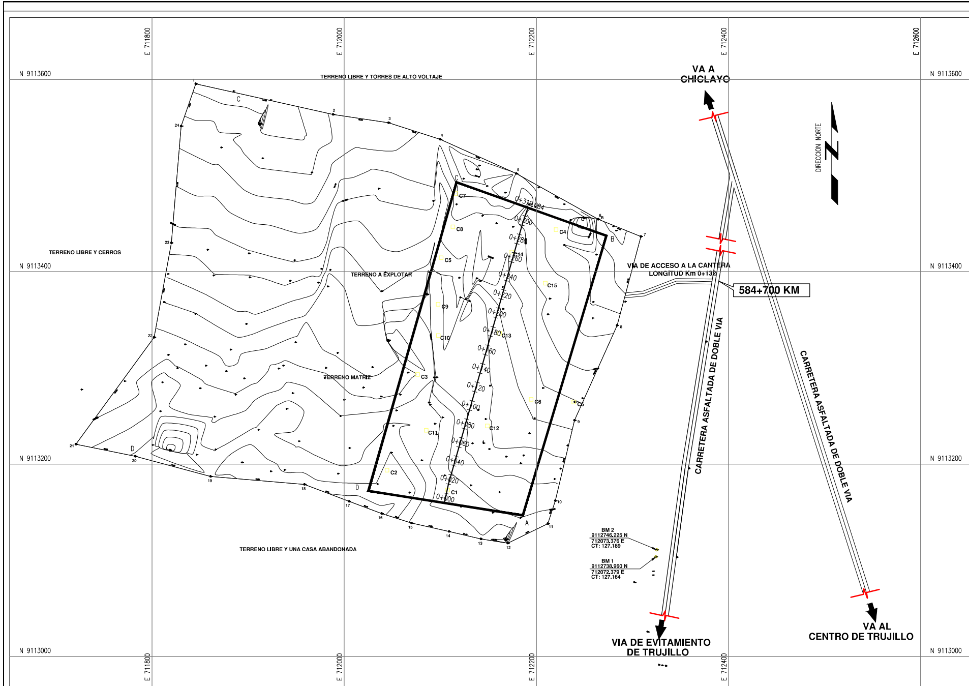
PLANTA 1:2000
