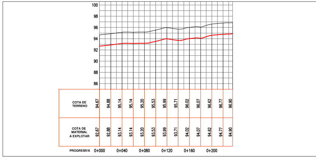
PERFIL H 1:2000 / V:1:200
