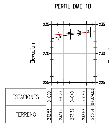
PERFIL ESC H 1:2000 / V 1:200
