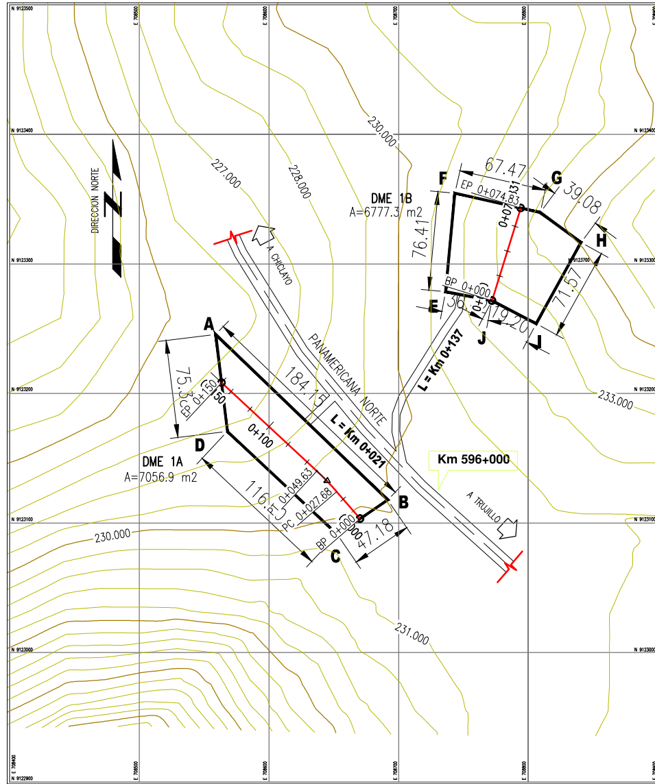
PLANTA ESC 1:2000
