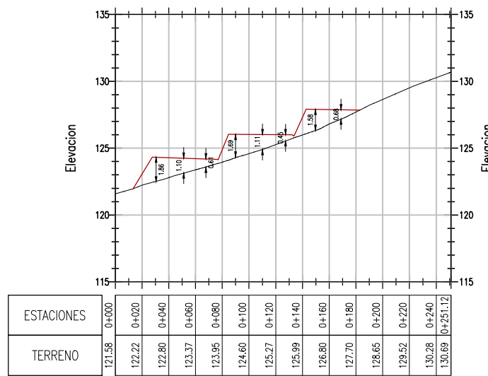
PERFIL ESC H 1:2000 / V 1:200
