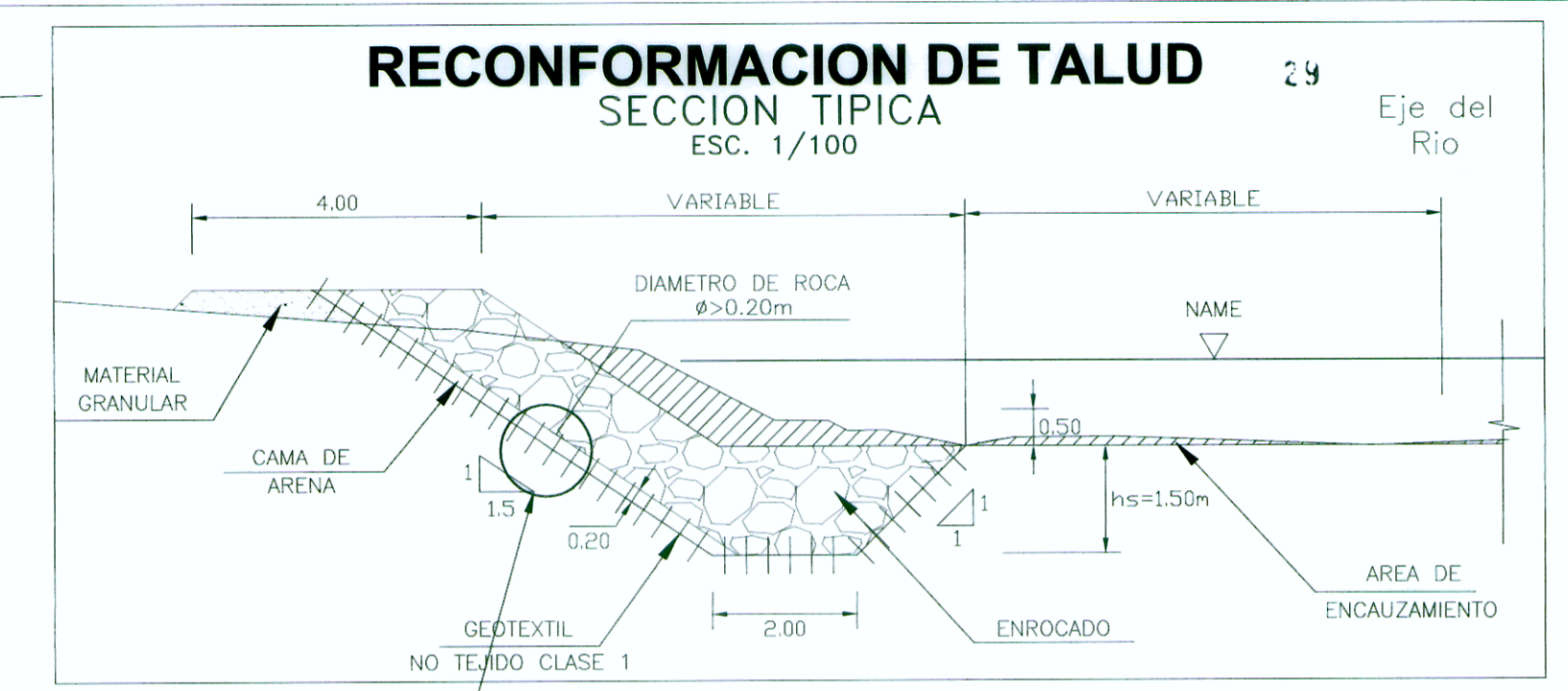
DETALLE 2
