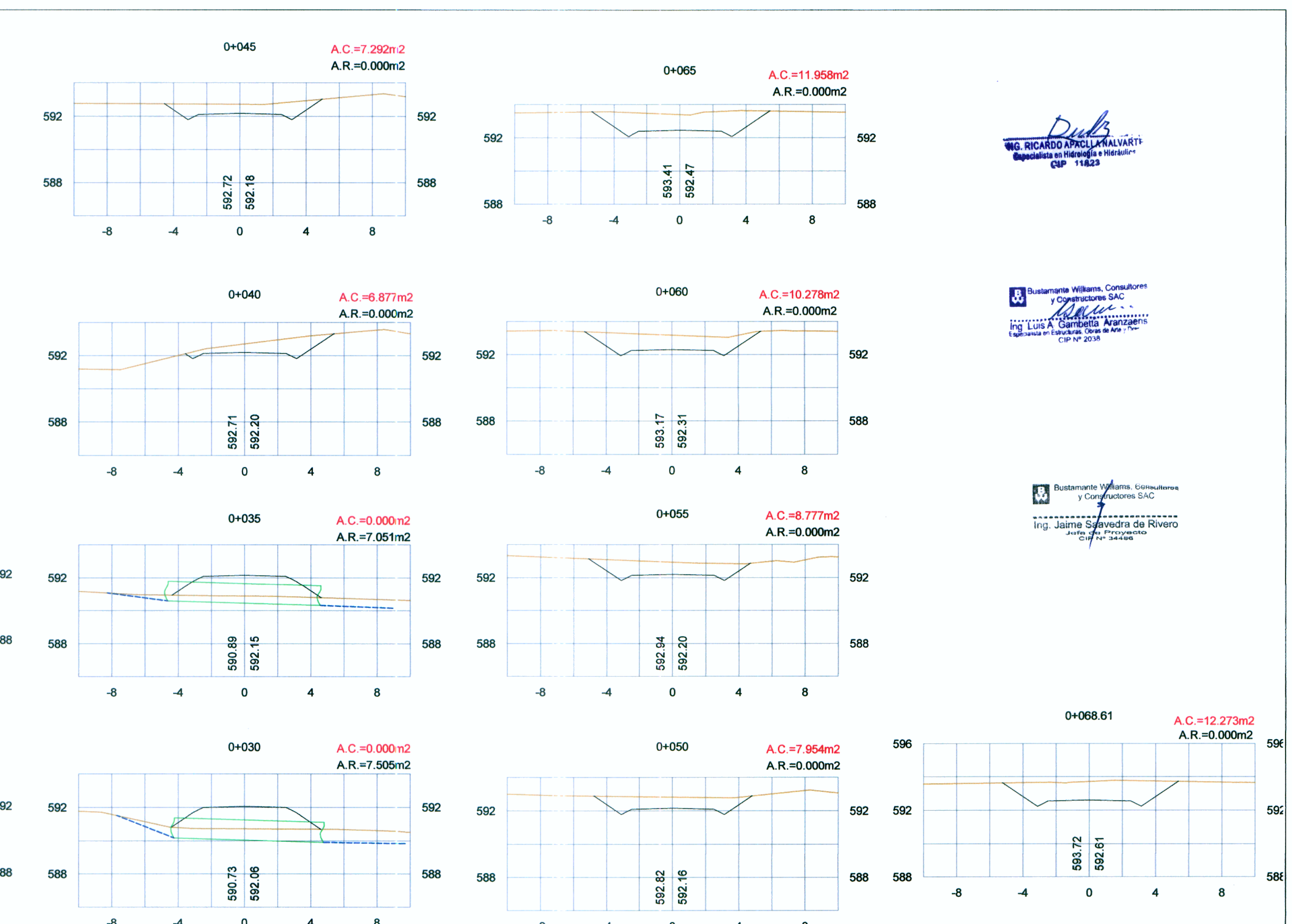
SECCIONES TRANSVERSALES ESCALA : 1/200
