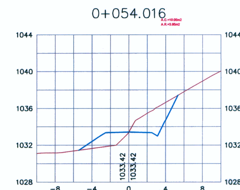
SECCIONES TRANSVERSALES ESCALA: 1/ 250
