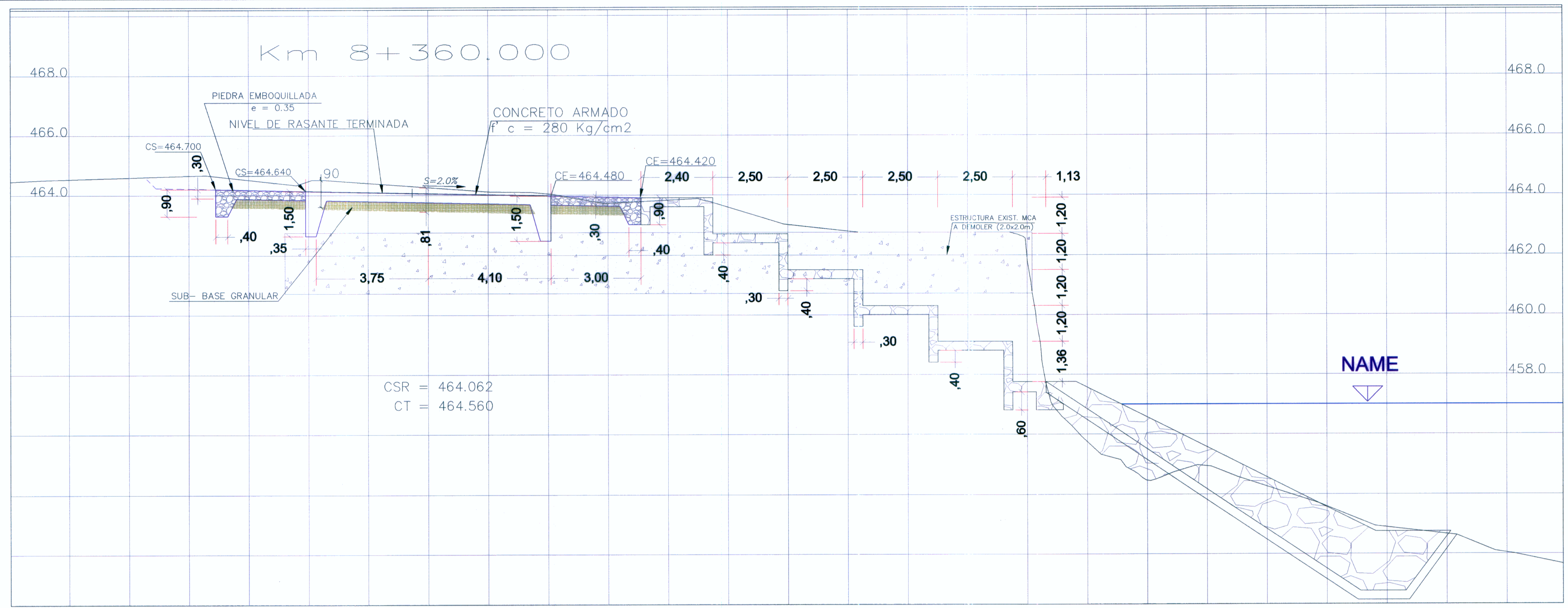
SECCION 1:100
