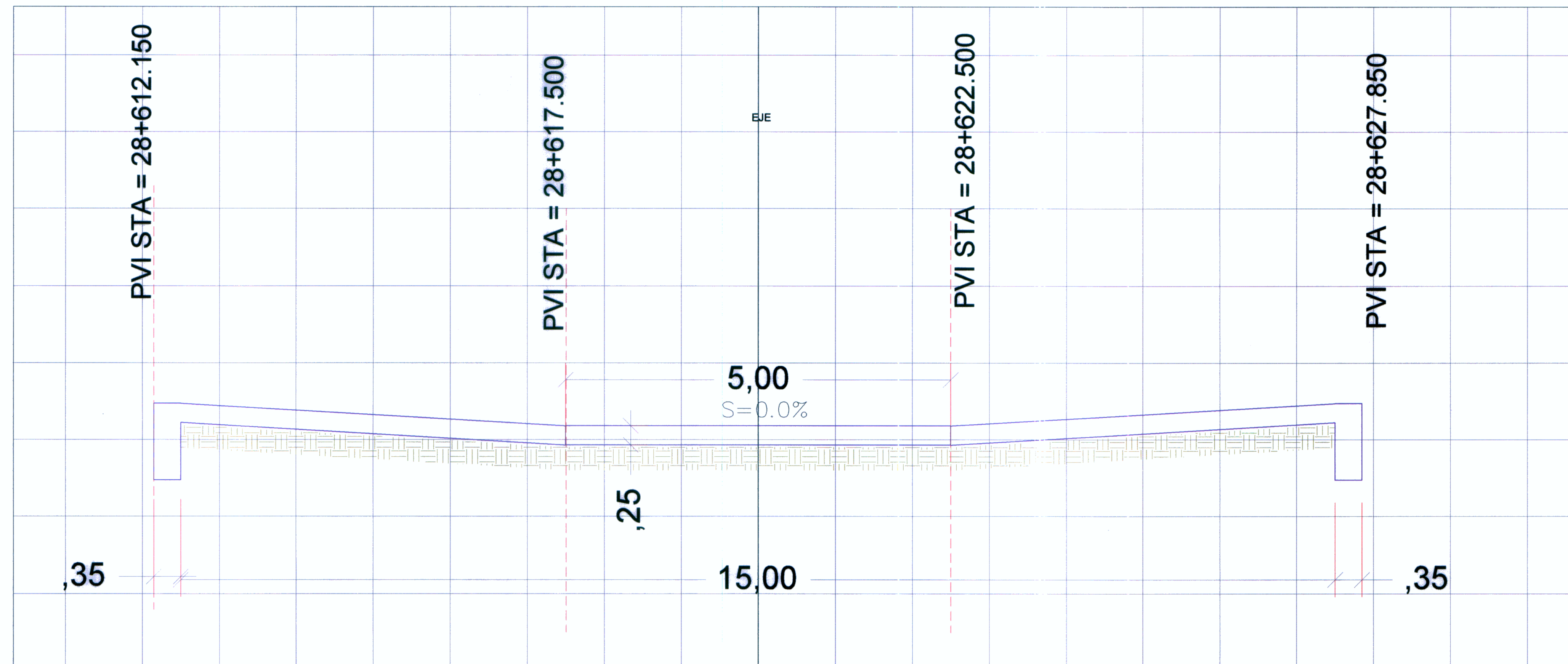
PERFIL 1:20
