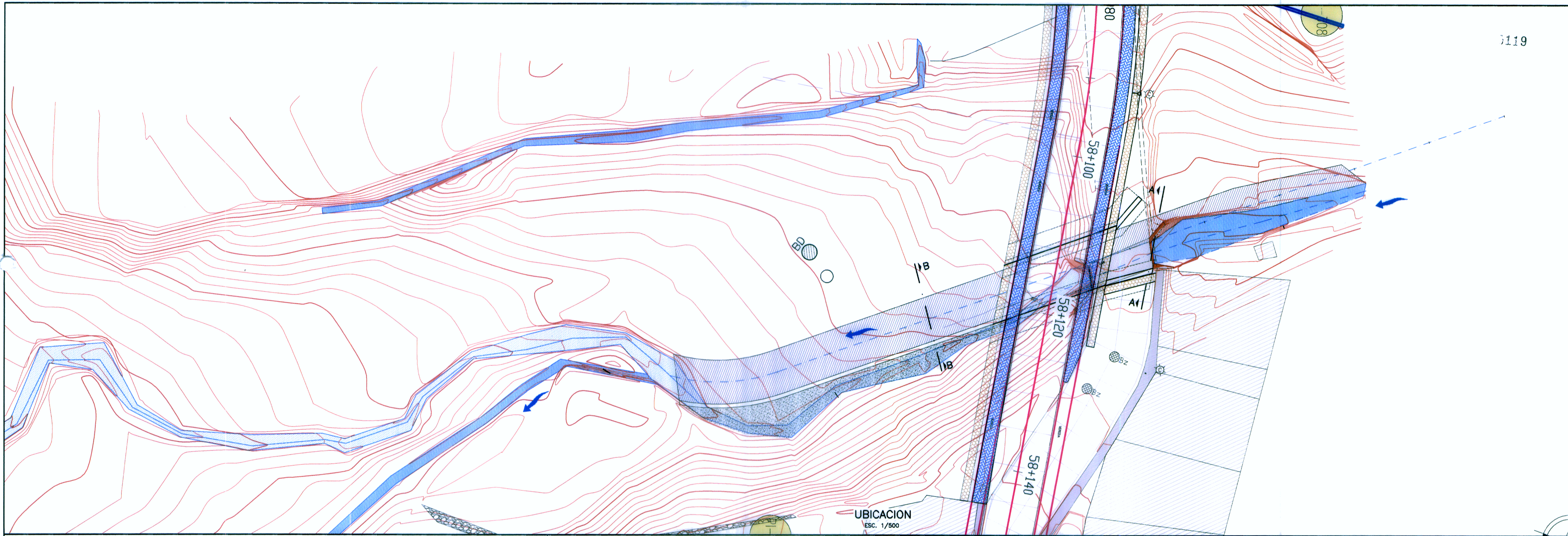
ALCANTARILLA PERFIL BAJO 6.50x2.36 ESVIAJADO 60° PROYECTAR 58+115
