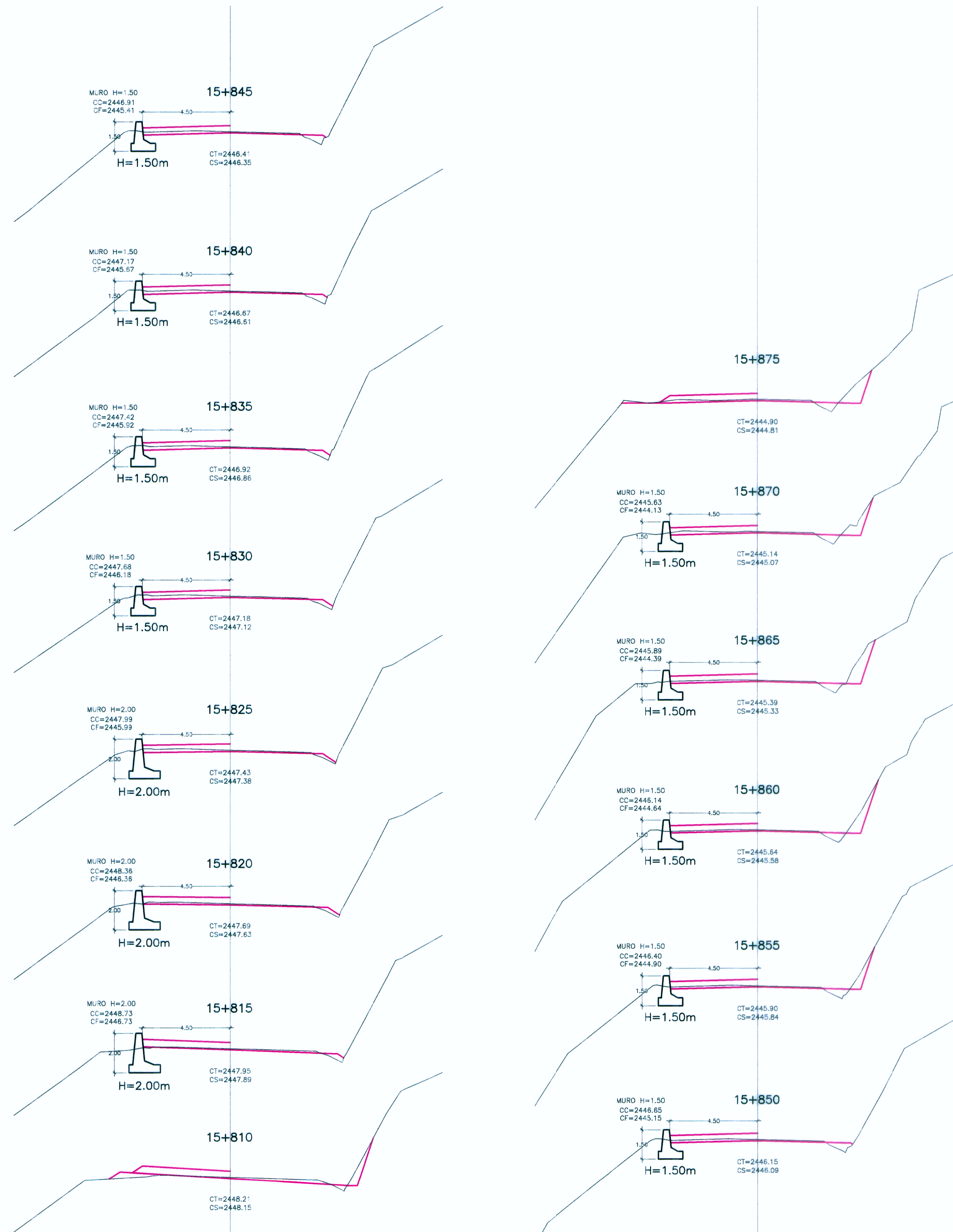
SECCIONES TRANSVERSALES ESC.: 1/125
